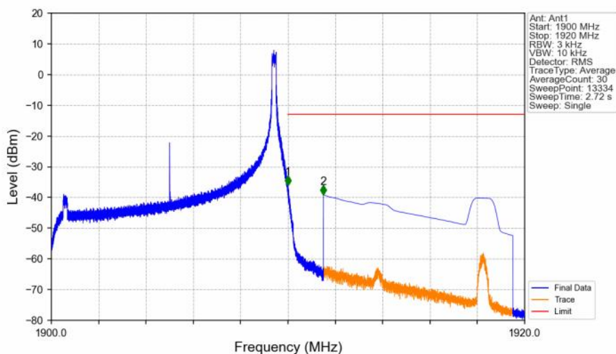
Band2_10MHz_16QAM_HCH_1905MHz_RB_1_49_NTNV
