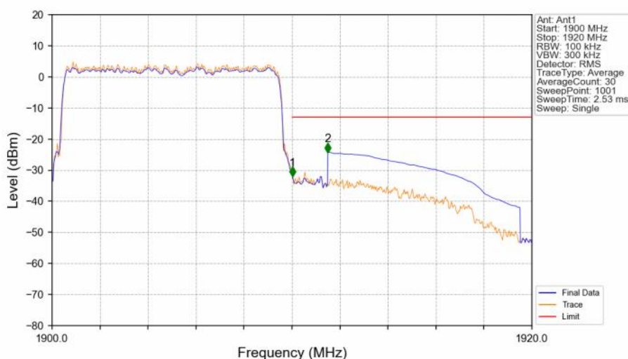
Band2_10MHz_16QAM_HCH_1905MHz_RB_50_0_NTNV
