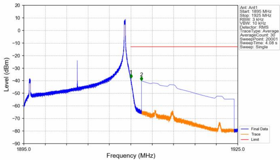
Band2_15MHz_QPSK_HCH_1902.5MHz_RB_1_74_NTNV
