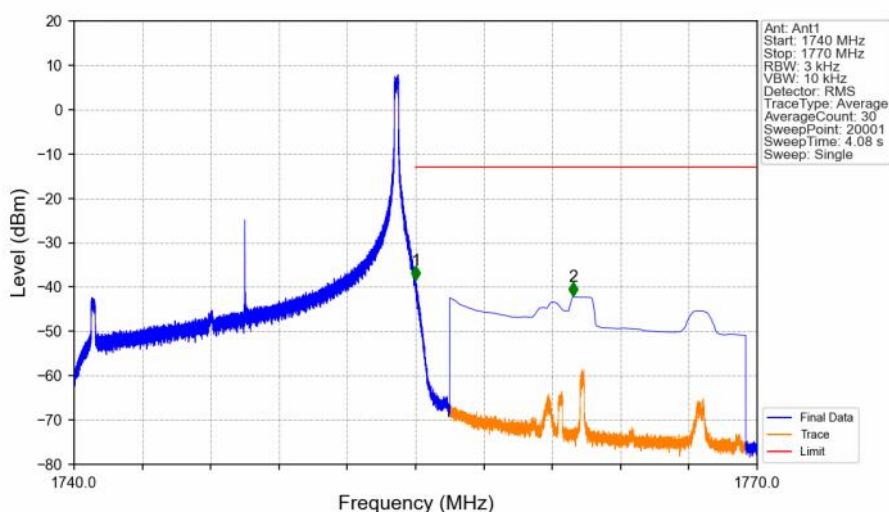
Band4_15MHz_QPSK_HCH_1747.5MHz_RB_1_74_NTNV
