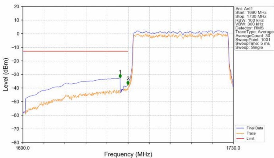
Band4_20MHz_16QAM_LCH_1720MHz_RB_100_0_NTNV
