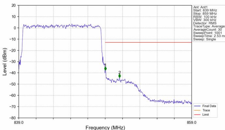
Band5_10MHz_QPSK_HCH_844MHz_RB_50_0_NTNV
