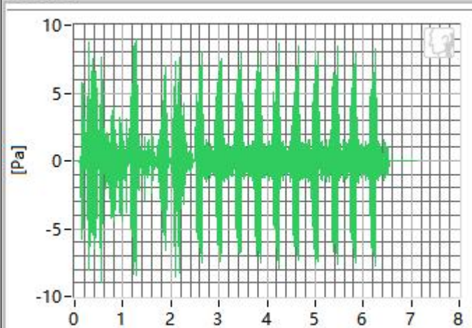
500Hz
