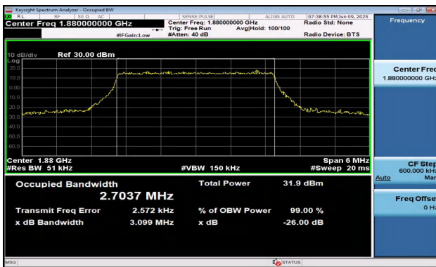
Band2-3MHz-QPSK-18900-15RB#0-PASS
