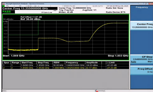
Band2-3MHz-16QAM-18615-1RB#14-PASS
