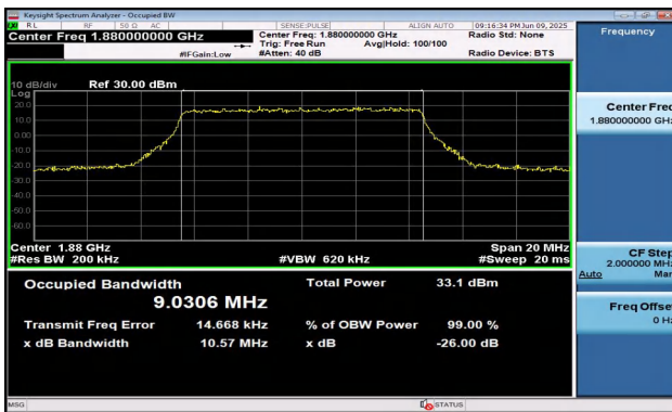
Band2-10MHz-QPSK-18900-50RB#0-PASS
