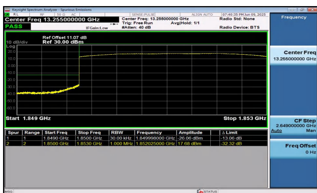
Band2-3MHz-QPSK-18615-15RB#0-PASS
