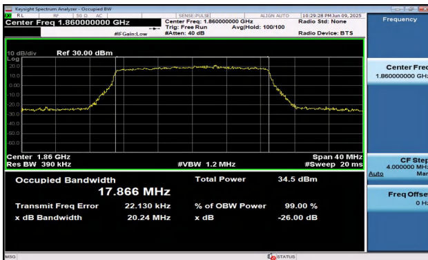
Band2-20MHz-QPSK-18700-100RB#0-PASS
