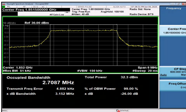
Band2-3MHz-QPSK-18615-15RB#0-PASS
