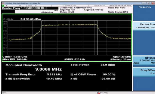
Band2-10MHz-QPSK-18650-50RB#0-PASS
