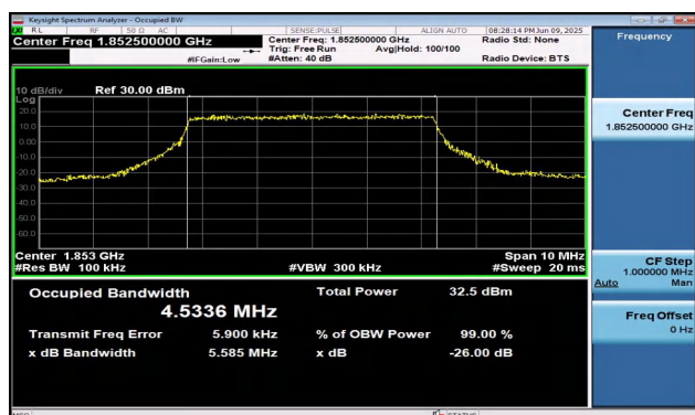
Band2-5MHz-QPSK-18625-25RB#0-PASS
