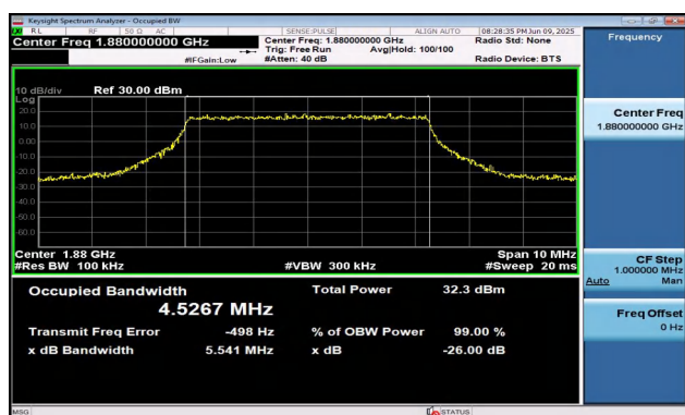
Band2-5MHz-QPSK-18900-25RB#0-PASS
