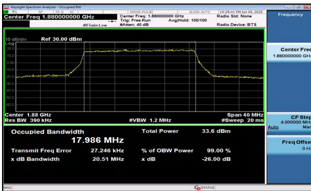
Band2-20MHz-QPSK-18900-100RB#0-PASS
