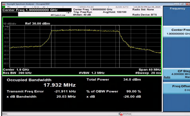
Band2-20MHz-QPSK-19100-100RB#0-PASS
