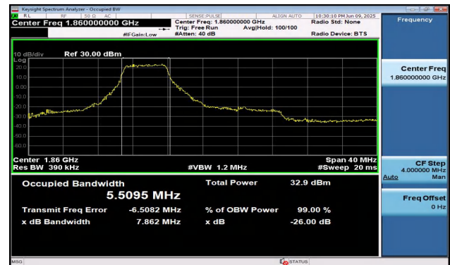
Band2-20MHz-16QAM-18700-27RB#0-PASS
