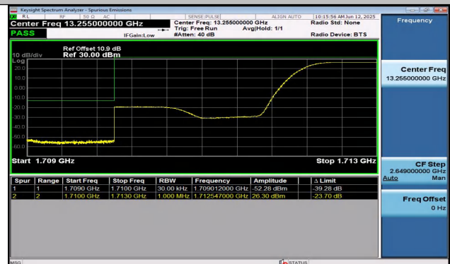
Band4-3MHz-QPSK-19965-1RB#14-PASS
