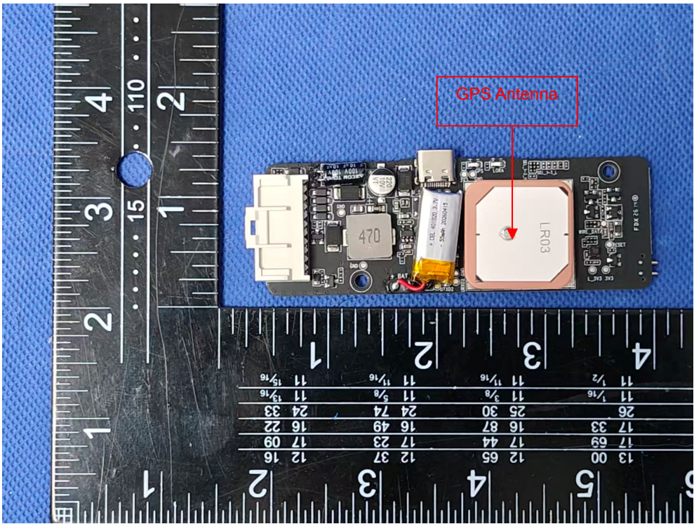
EUT Photo
