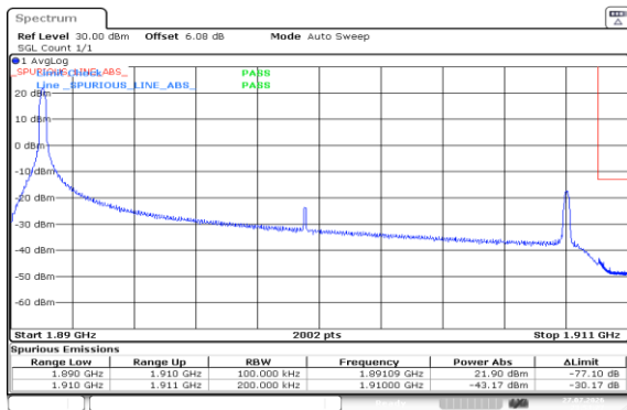
Band2-20MHz-QPSK-19100-1RB#0-PASS
