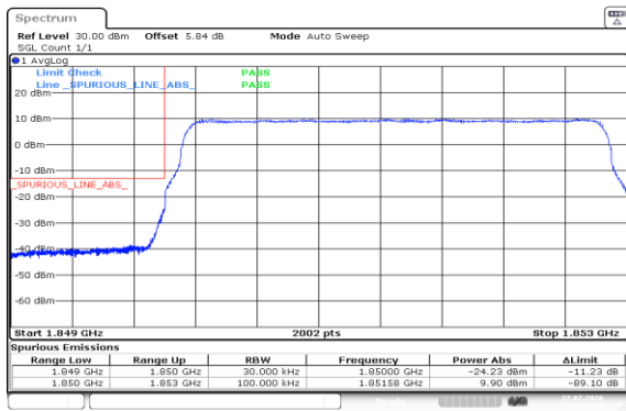
Band2-3MHz-QPSK-18615-15RB#0-PASS
