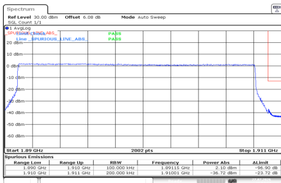
Band2-20MHz-QPSK-19100-100RB#0-PASS
