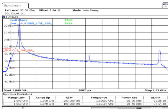
Band2-20MHz-QPSK-18700-1RB#0-PASS
