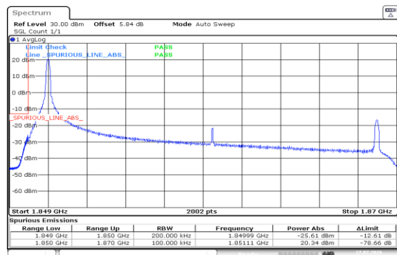
Band2-20MHz-16QAM-18700-1RB#0-PASS
