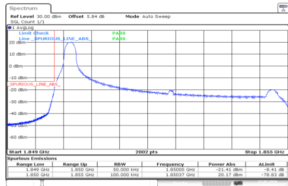
Band2-5MHz-16QAM-18625-1RB#0-PASS
