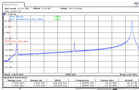
Band2-20MHz-16QAM-18700-1RB#99-PASS
