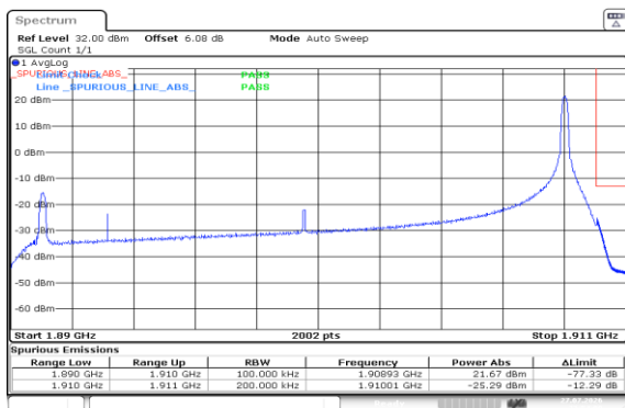
Band2-20MHz-QPSK-19100-1RB#99-PASS
