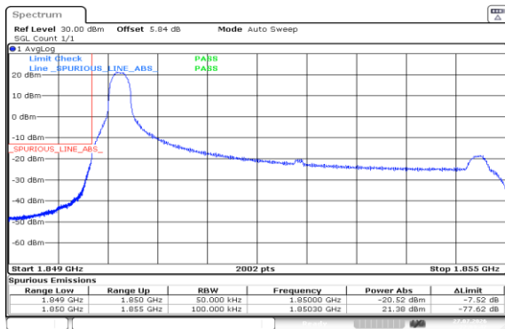
Band2-5MHz-QPSK-18625-1RB#0-PASS
