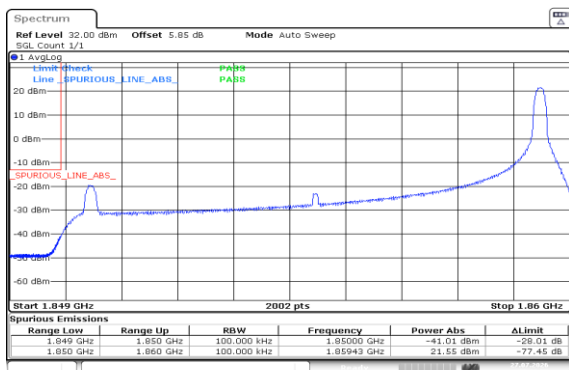
Band2-10MHz-QPSK-18650-1RB#49-PASS
