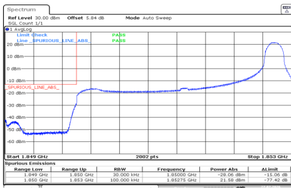
Band2-3MHz-QPSK-18615-1RB#14-PASS
