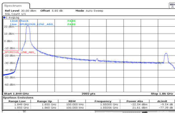
Band2-10MHz-QPSK-18650-1RB#0-PASS
