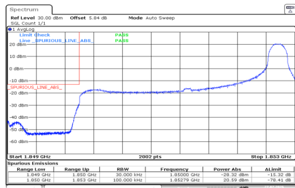
Band2-3MHz-16QAM-18615-1RB#14-PASS
