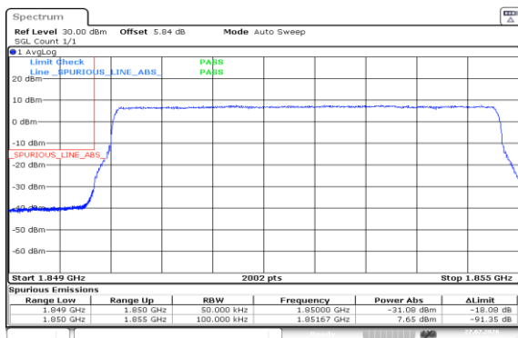
Band2-5MHz-QPSK-18625-25RB#0-PASS
