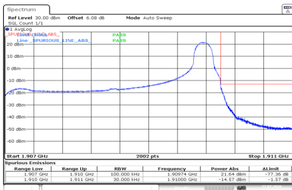
Band2-3MHz-QPSK-19185-1RB#14-PASS
