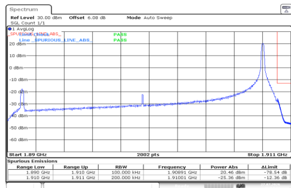
Band2-20MHz-16QAM-19100-1RB#99-PASS
