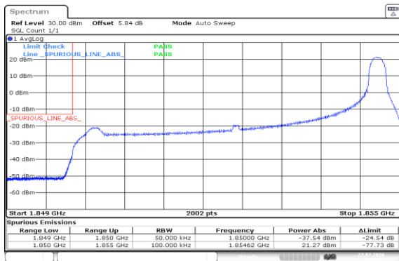
Band2-5MHz-QPSK-18625-1RB#24-PASS
