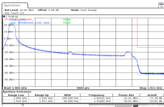
Band2-5MHz-QPSK-19175-1RB#0-PASS
