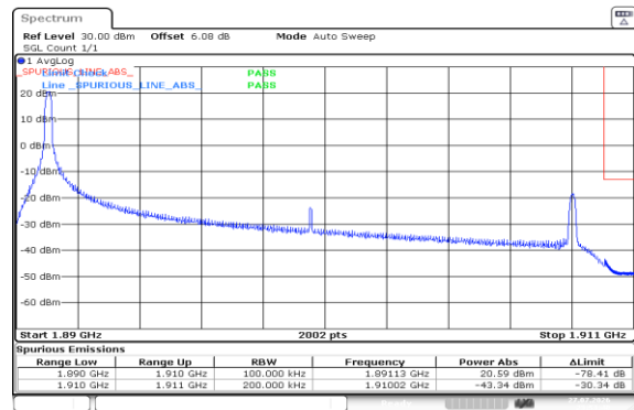
Band2-20MHz-16QAM-19100-1RB#0-PASS
