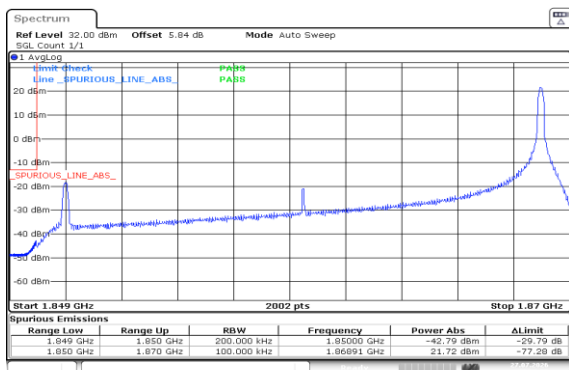
Band2-20MHz-QPSK-18700-1RB#99-PASS
