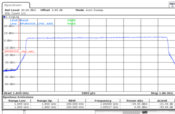
Band2-10MHz-QPSK-18650-50RB#0-PASS
