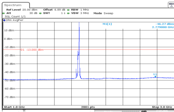
Band2-20MHz-QPSK-18900-1RB#99-1000~3000-PASS
