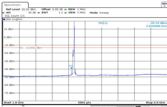
Band2-20MHz-QPSK-18700-1RB#99-1000~3000-PASS
