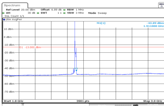
Band2-20MHz-QPSK-19100-1RB#0-1000~3000-PASS
