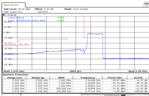
Band38-20MHz-QPSK-37850-1RB#99-PASS
