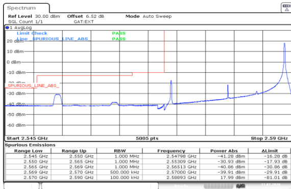
Band38-20MHz-QPSK-37850-1RB#99-PASS
