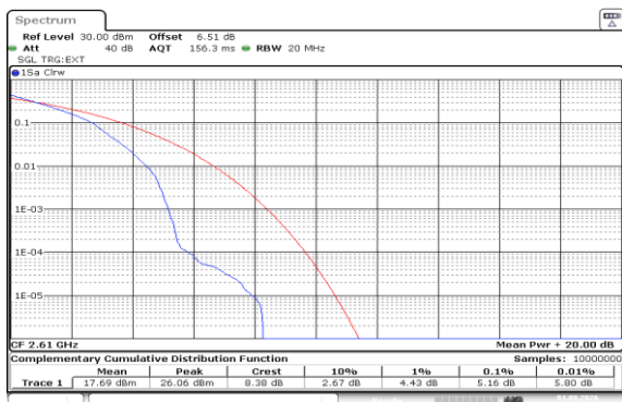
Band38-20MHz-QPSK-38150-1RB#0-PASS
