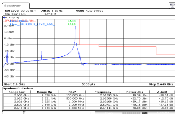
Band38-20MHz-QPSK-38150-1RB#99-PASS
