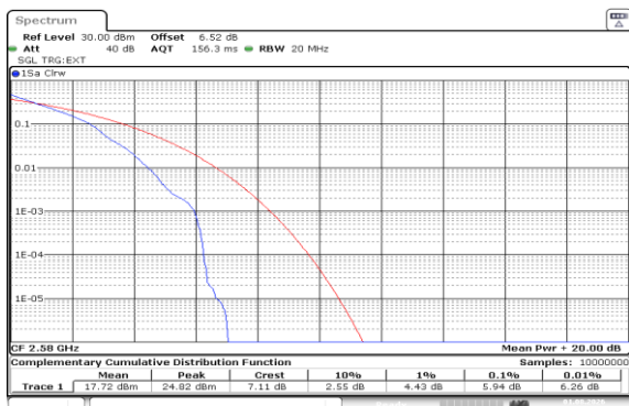
Band38-20MHz-QPSK-37850-1RB#0-PASS
