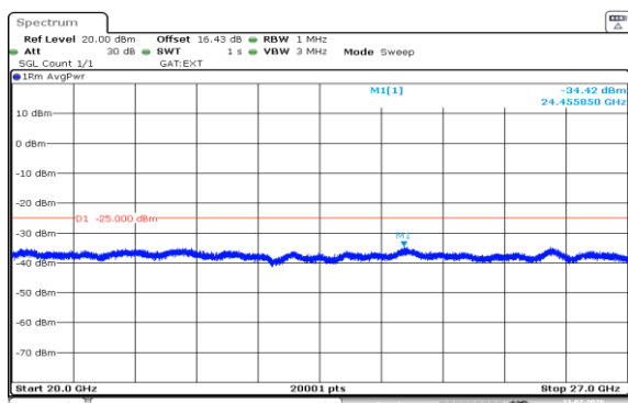
Band38-5MHz-QPSK-38000-25RB#0-20000~27000-PASS
