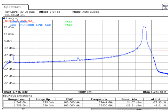
Band4-10MHz-QPSK-20350-1RB#49-PASS
