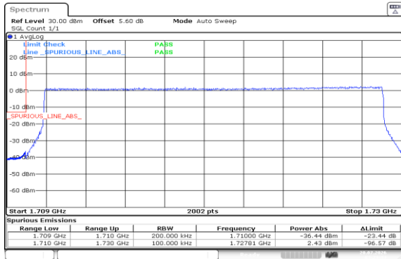
Band4-20MHz-QPSK-20050-100RB#0-PASS
