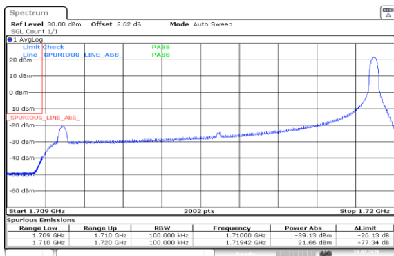
Band4-10MHz-QPSK-20000-1RB#49-PASS
