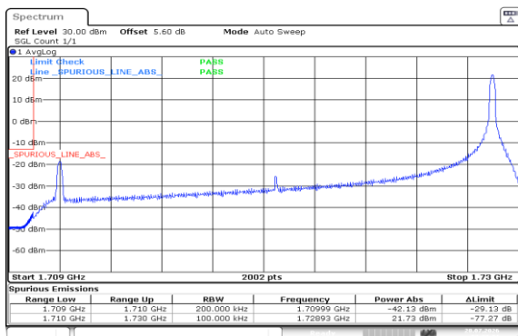
Band4-20MHz-QPSK-20050-1RB#99-PASS
