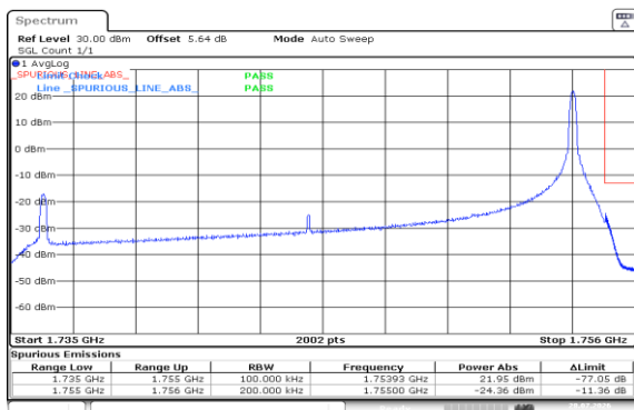
Band4-20MHz-QPSK-20300-1RB#99-PASS
