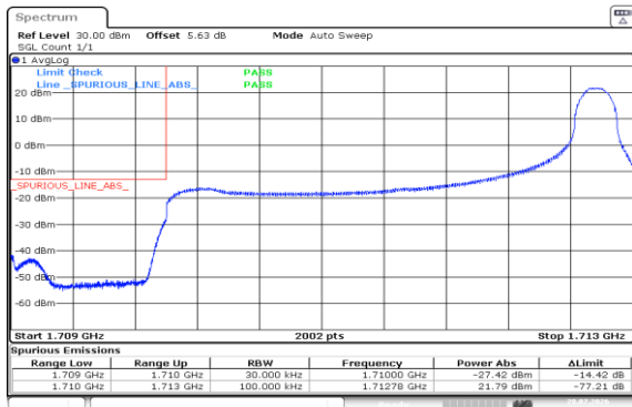
Band4-3MHz-QPSK-19965-1RB#14-PASS
