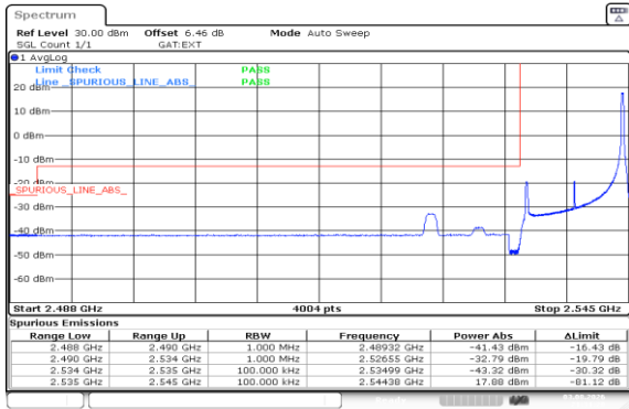
Band41(2535-2655)-10MHz-QPSK-40090-1RB#49-PASS
