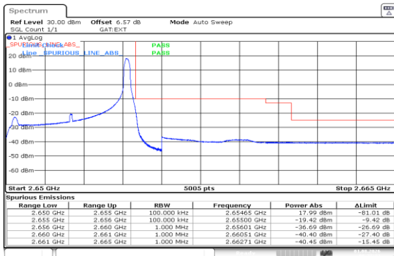
Band41(2535-2655)-5MHz-QPSK-41215-1RB#24-PASS
