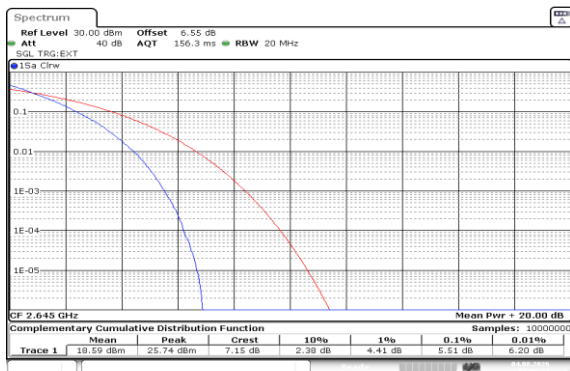
Band41(2535-2655)-20MHz-QPSK-41140-100RB#0-PASS
