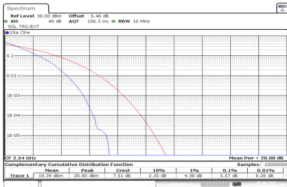
Band41(2535-2655)-10MHz-QPSK-40090-50RB#0-PASS
