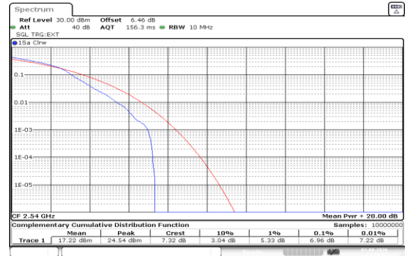
Band41(2535-2655)-10MHz-16QAM-40090-1RB#0-PASS
