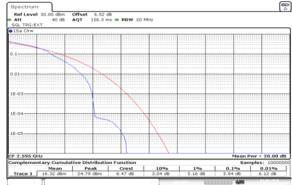
Band41(2535-2655)-20MHz-16QAM-40640-1RB#0-PASS
