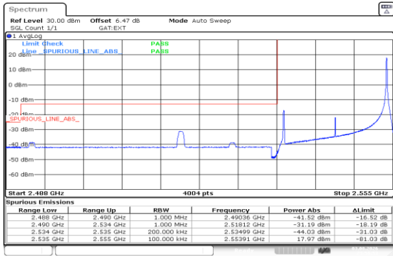
Band41(2535-2655)-20MHz-QPSK-40140-1RB#99-PASS
