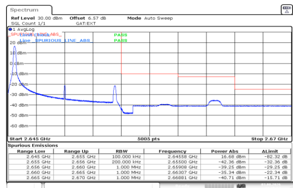
Band41(2535-2655)-10MHz-16QAM-41190-1RB#0-PASS
