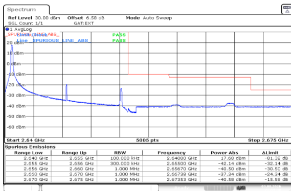
Band41(2535-2655)-15MHz-QPSK-41165-1RB#0-PASS
