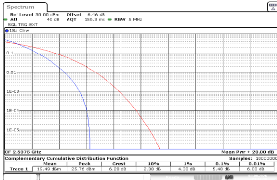
Band41(2535-2655)-5MHz-QPSK-40065-25RB#0-PASS
