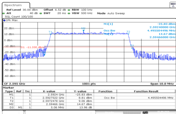
Band41(2535-2655)-5MHz-QPSK-40640-25RB#0-PASS
