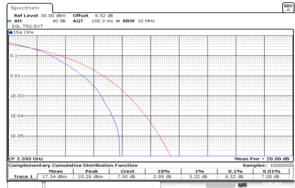
Band41(2535-2655)-10MHz-16QAM-40640-50RB#0-PASS
