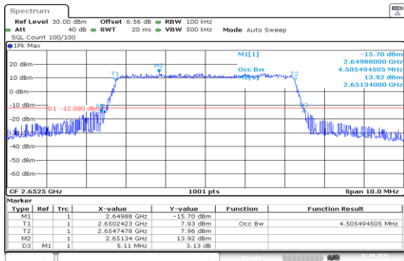
Band41(2535-2655)-5MHz-QPSK-41215-25RB#0-PASS
