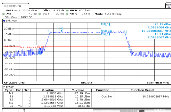
Band41(2535-2655)-20MHz-QPSK-40640-100RB#0-PASS
