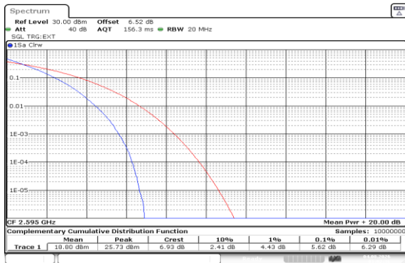
Band41(2535-2655)-20MHz-QPSK-40640-100RB#0-PASS
