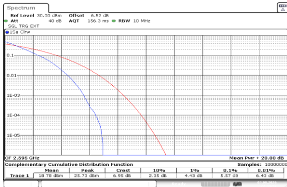
Band41(2535-2655)-10MHz-QPSK-40640-50RB#0-PASS
