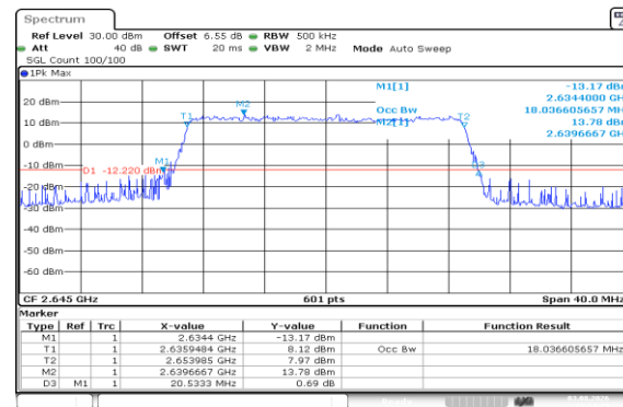
Band41(2535-2655)-20MHz-QPSK-41140-100RB#0-PASS
