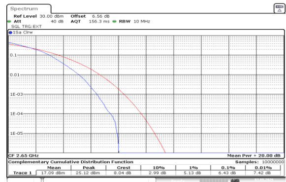
Band41(2535-2655)-10MHz-16QAM-41190-50RB#0-PASS
