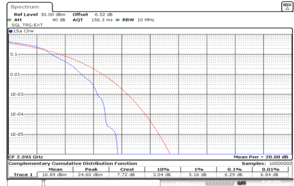
Band41(2535-2655)-10MHz-16QAM-40640-1RB#0-PASS
