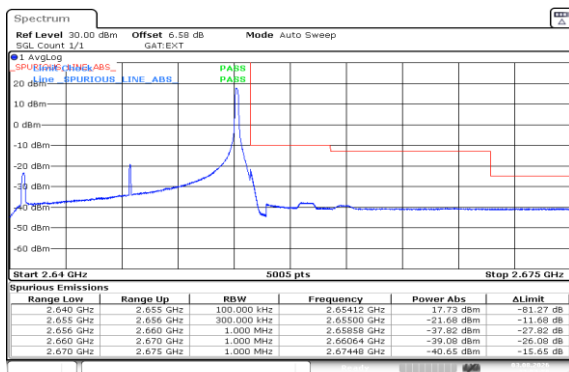
Band41(2535-2655)-15MHz-QPSK-41165-1RB#74-PASS
