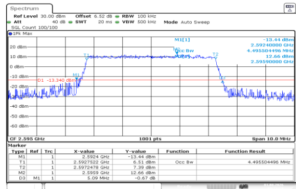
Band41(2535-2655)-5MHz-16QAM-40640-25RB#0-PASS
