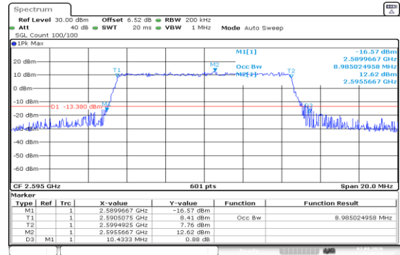
Band41(2535-2655)-10MHz-16QAM-40640-50RB#0-PASS
