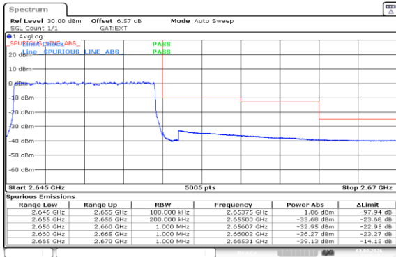
Band41(2535-2655)-10MHz-QPSK-41190-50RB#0-PASS
