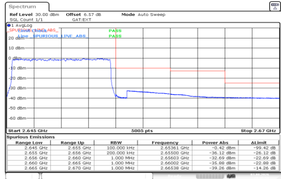
Band41(2535-2655)-10MHz-16QAM-41190-50RB#0-PASS
