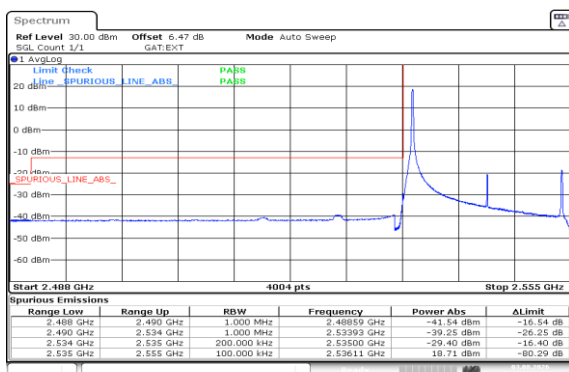
Band41(2535-2655)-20MHz-QPSK-40140-1RB#0-PASS
