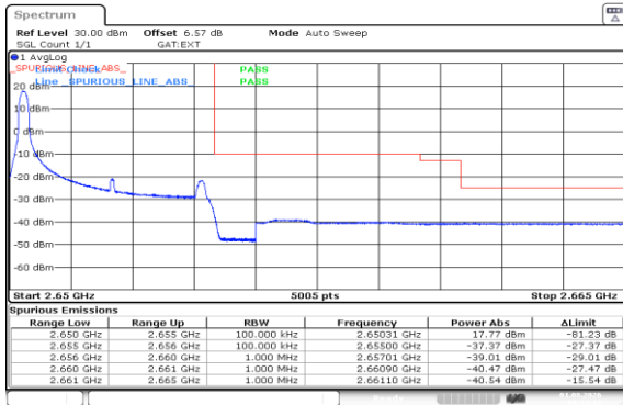
Band41(2535-2655)-5MHz-QPSK-41215-1RB#0-PASS
