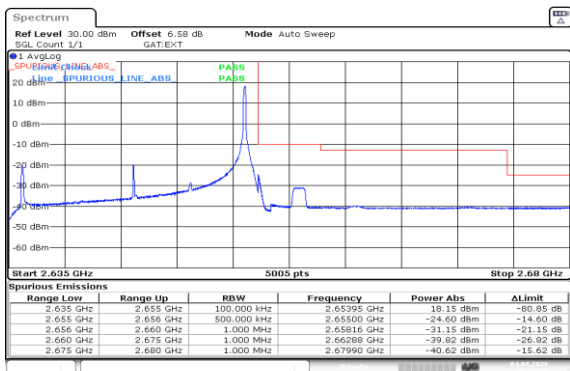
Band41(2535-2655)-20MHz-QPSK-41140-1RB#99-PASS
