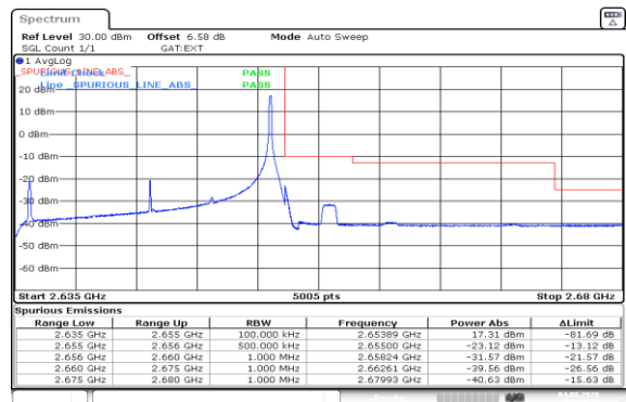
Band41(2535-2655)-20MHz-16QAM-41140-1RB#99-PASS
