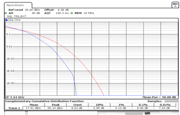
Band41(2535-2655)-10MHz-16QAM-40090-50RB#0-PASS
