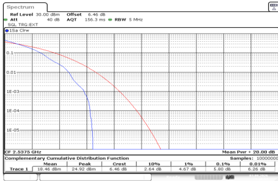
Band41(2535-2655)-5MHz-QPSK-40065-1RB#0-PASS
