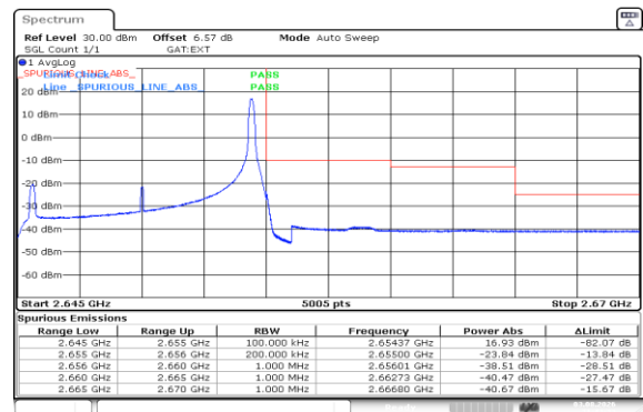
Band41(2535-2655)-10MHz-16QAM-41190-1RB#49-PASS
