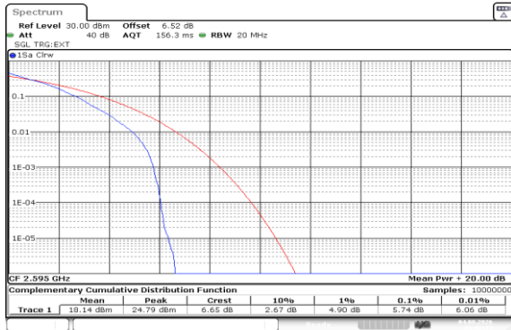
Band41(2535-2655)-20MHz-QPSK-40640-1RB#0-PASS
