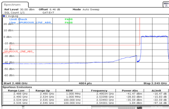
Band41(2535-2655)-10MHz-QPSK-40090-50RB#0-PASS
