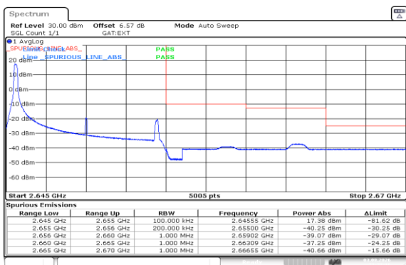
Band41(2535-2655)-10MHz-QPSK-41190-1RB#0-PASS
