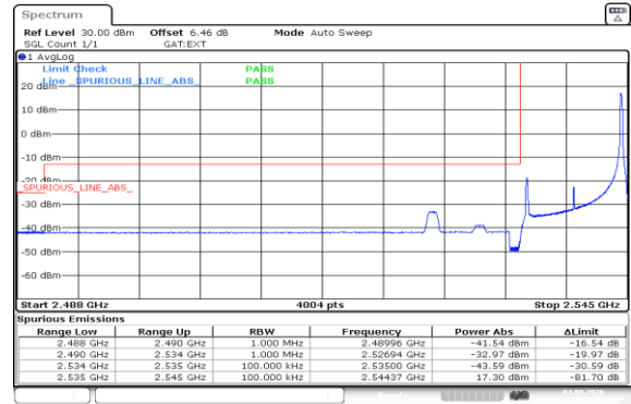
Band41(2535-2655)-10MHz-16QAM-40090-1RB#49-PASS
