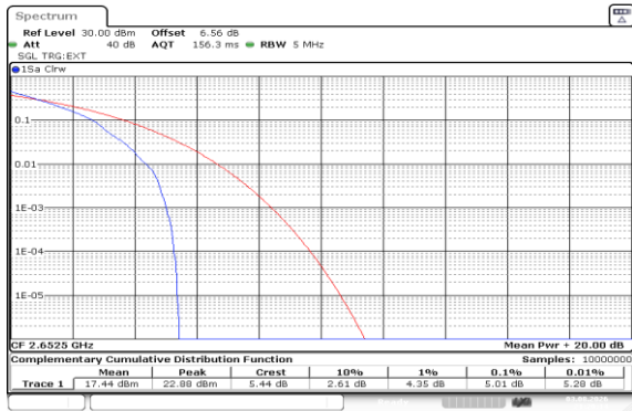
Band41(2535-2655)-5MHz-QPSK-41215-1RB#0-PASS
