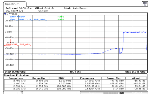
Band41(2535-2655)-10MHz-16QAM-40090-50RB#0-PASS
