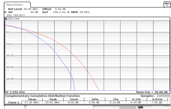
Band41(2535-2655)-20MHz-16QAM-40640-100RB#0-PASS
