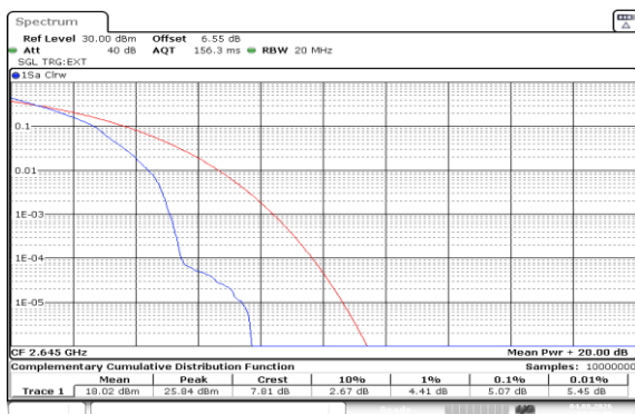
Band41(2535-2655)-20MHz-QPSK-41140-1RB#0-PASS
