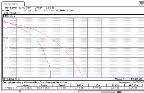
Band41(2535-2655)-5MHz-QPSK-40640-1RB#0-PASS
