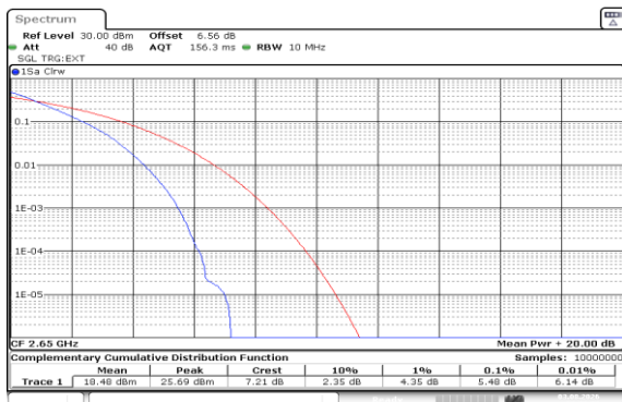
Band41(2535-2655)-10MHz-QPSK-41190-50RB#0-PASS
