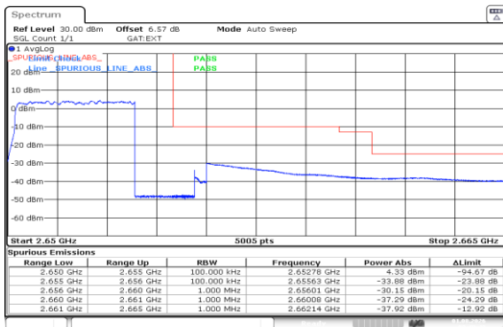
Band41(2535-2655)-5MHz-QPSK-41215-25RB#0-PASS
