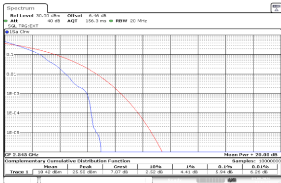
Band41(2535-2655)-20MHz-QPSK-40140-1RB#0-PASS
