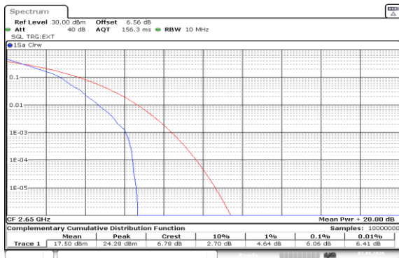
Band41(2535-2655)-10MHz-QPSK-41190-1RB#0-PASS
