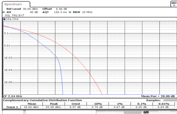
Band41(2535-2655)-10MHz-QPSK-40090-1RB#0-PASS
