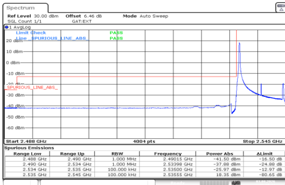
Band41(2535-2655)-10MHz-QPSK-40090-1RB#0-PASS
