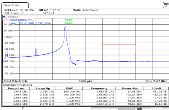
Band41(2535-2655)-10MHz-QPSK-41190-1RB#49-PASS
