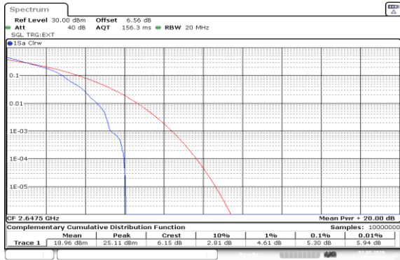
Band41(2535-2655)-15MHz-QPSK-41165-1RB#0-PASS
