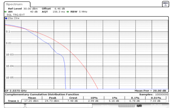
Band41(2535-2655)-5MHz-16QAM-40065-1RB#0-PASS
