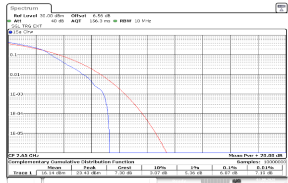
Band41(2535-2655)-10MHz-16QAM-41190-1RB#0-PASS
