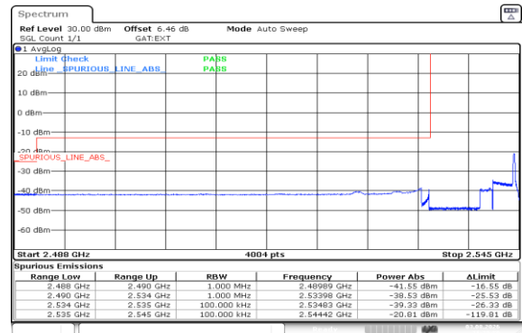
Band41(2535-2655)-10MHz-16QAM-40090-1RB#0-PASS
