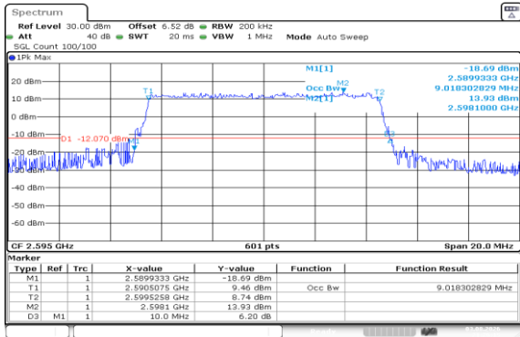
Band41(2535-2655)-10MHz-QPSK-40640-50RB#0-PASS
