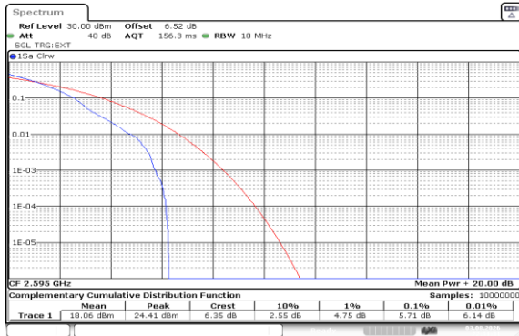
Band41(2535-2655)-10MHz-QPSK-40640-1RB#0-PASS
