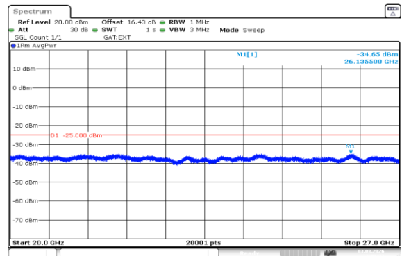
Band41(2535-2655)-10MHz-16QAM-40640-1RB#0-20000~27000-PASS
