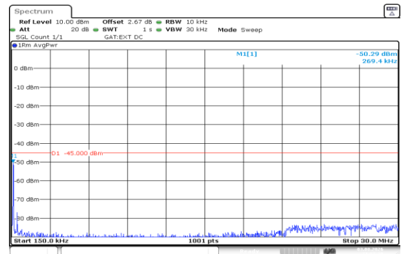
Band41(2535-2655)-10MHz-QPSK-40640-1RB#0-0.15~30-PASS
