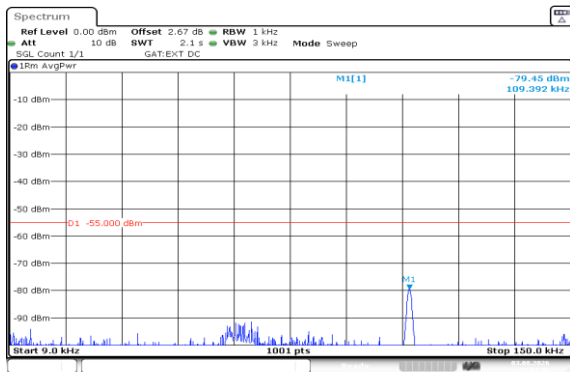
Band41(2535-2655)-10MHz-QPSK-40640-50RB#0-0.009~0.15-PASS
