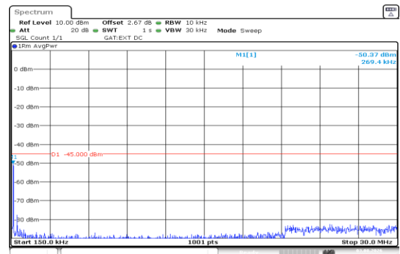
Band41(2535-2655)-10MHz-QPSK-41190-50RB#0-0.15~30-PASS
