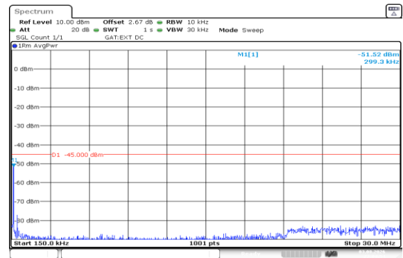
Band41(2535-2655)-10MHz-QPSK-40640-50RB#0-0.15~30-PASS
