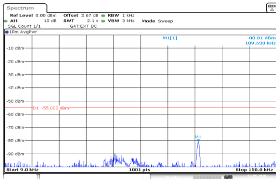
Band41(2535-2655)-10MHz-QPSK-40640-1RB#0-0.009~0.15-PASS
