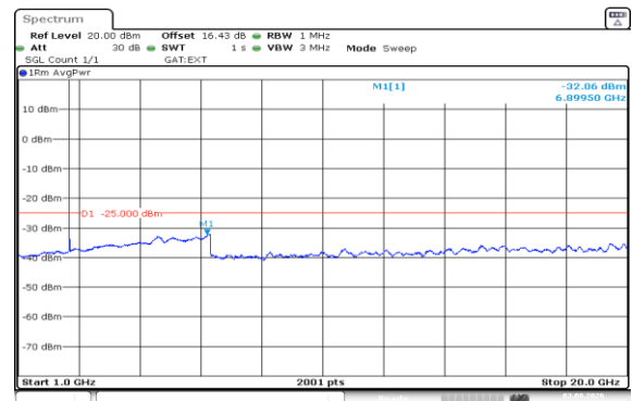
Band41(2535-2655)-10MHz-QPSK-40640-1RB#0-1000~20000-PASS
