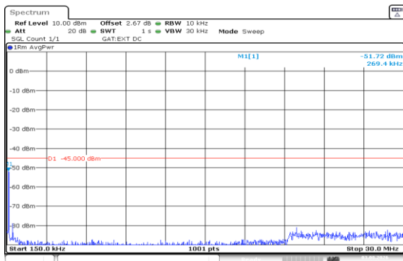
Band41(2535-2655)-10MHz-16QAM-40640-50RB#0-0.15~30-PASS
