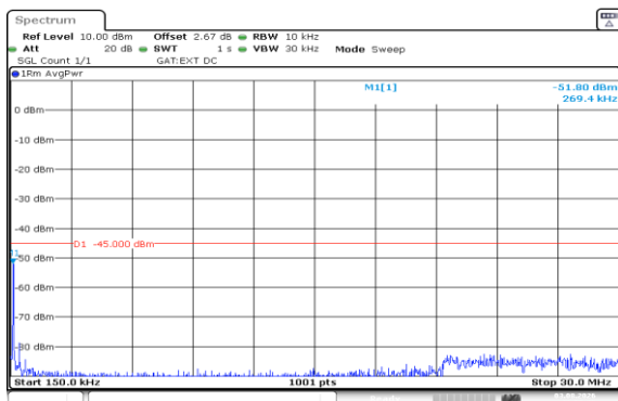
Band41(2535-2655)-10MHz-QPSK-40640-1RB#0-20000-PASS
