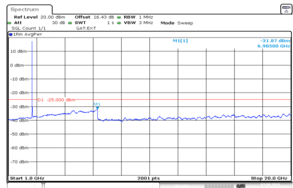
Band41(2535-2655)-10MHz-QPSK-40640-50RB#0-1000~20000-PASS
