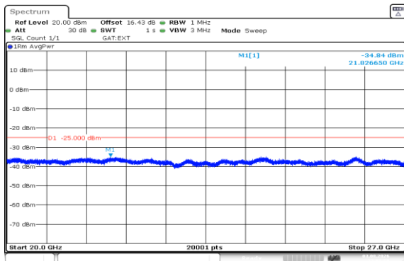
Band41(2535-2655)-10MHz-QPSK-40640-50RB#0-20000~27000-PASS
