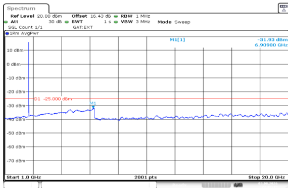
Band41(2535-2655)-10MHz-16QAM-40640-50RB#0-1000~20000-PASS
