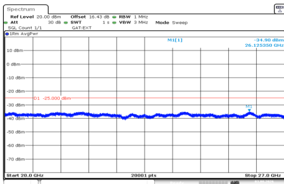
Band41(2535-2655)-10MHz-QPSK-41190-50RB#0-20000~27000-PASS
