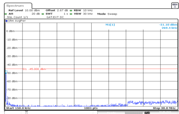
Band41(2535-2655)-10MHz-QPSK-41190-1RB#0-0.15~30-PASS
