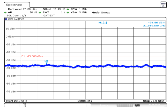
Band41(2535-2655)-10MHz-16QAM-40640-50RB#0-20000~27000-PASS
