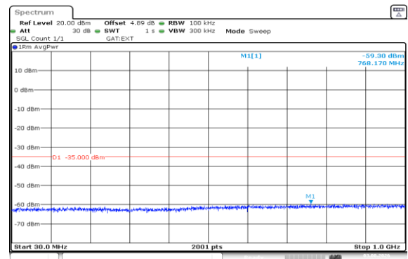
Band41(2535-2655)-10MHz-16QAM-40640-50RB#0-30~1000-PASS
