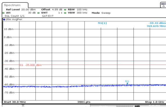
Band41(2535-2655)-10MHz-QPSK-40640-1RB#0-30~1000-PASS
