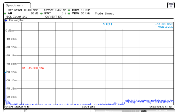
Band41(2535-2655)-10MHz-QPSK-40640-1RB#49-0.15~30-PASS
