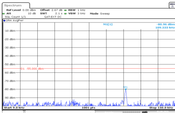
Band41(2535-2655)-10MHz-QPSK-40640-1RB#49-0.009~0.15-PASS
