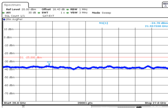
Band41(2535-2655)-5MHz-QPSK-41215-1RB#0-20000~27000-PASS
