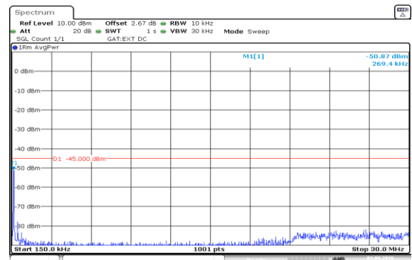
Band41(2535-2655)-10MHz-QPSK-40090-1RB#0-0.15~30-PASS
