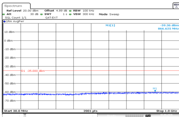
Band41(2535-2655)-10MHz-QPSK-40640-50RB#0-30~1000-PASS
