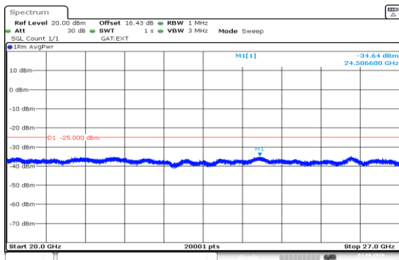
Band41(2535-2655)-10MHz-QPSK-41190-1RB#0-20000~27000-PASS
