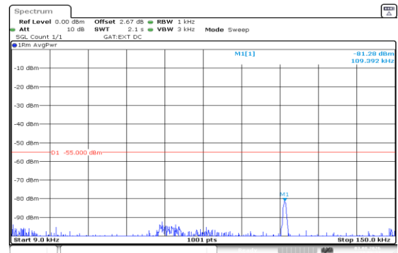
Band41(2535-2655)-10MHz-16QAM-40640-50RB#0-0.009~0.15-PASS
