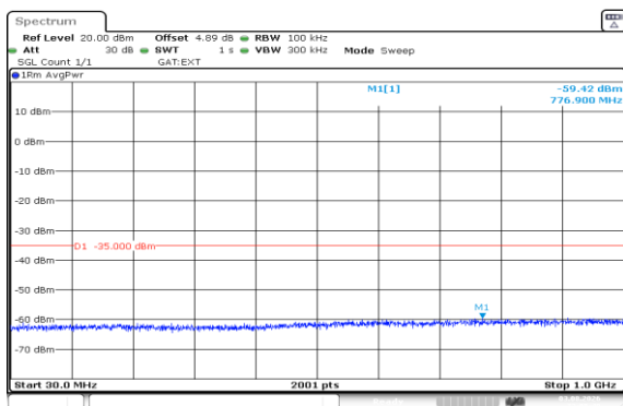
Band41(2535-2655)-10MHz-QPSK-41190-1RB#0-30~1000-PASS
