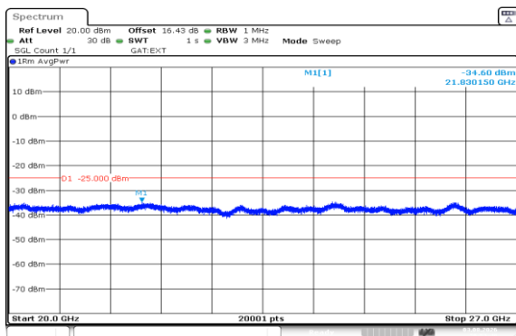
Band41(2535-2655)-5MHz-QPSK-40640-25RB#0-20000~27000-PASS
