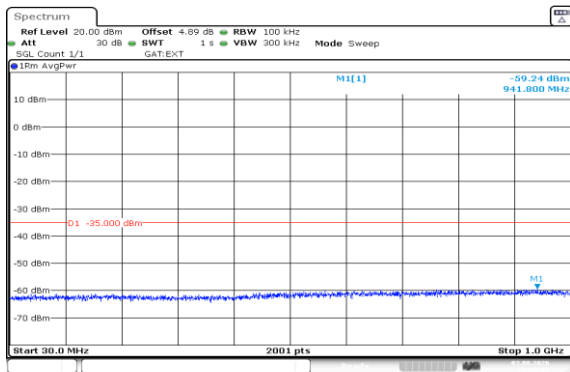
Band41(2535-2655)-10MHz-QPSK-41190-50RB#0-30~1000-PASS
