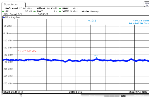
Band41(2535-2655)-5MHz-QPSK-40065-1RB#0-20000~27000-PASS
