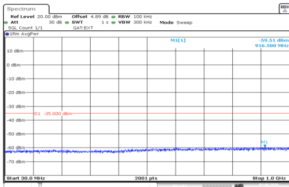
Band41(2535-2655)-10MHz-QPSK-41190-1RB#49-30~1000-PASS
