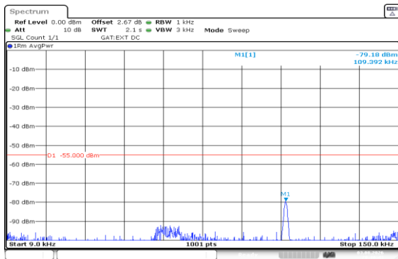
Band41(2535-2655)-5MHz-QPSK-40065-25RB#0-0.009~0.15-PASS
