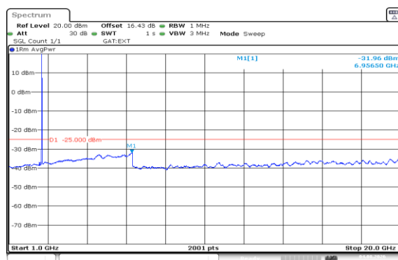
Band41(2535-2655)-20MHz-QPSK-40640-1RB#99-1000~20000-PASS
