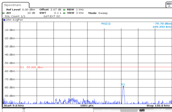
Band41(2535-2655)-20MHz-QPSK-40640-1RB#0-0.009~0.15-PASS
