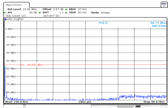
Band41(2535-2655)-20MHz-QPSK-40640-1RB#0-0.15~30-PASS
