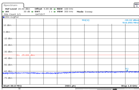
Band41(2535-2655)-20MHz-QPSK-40640-1RB#99-30~1000-PASS
