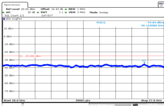
Band41(2535-2655)-20MHz-QPSK-40640-1RB#0-20000~27000-PASS
