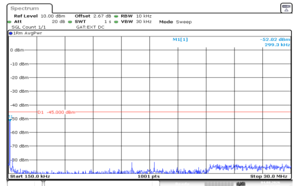
Band41(2535-2655)-20MHz-QPSK-40640-100RB#0-0.15~30-PASS
