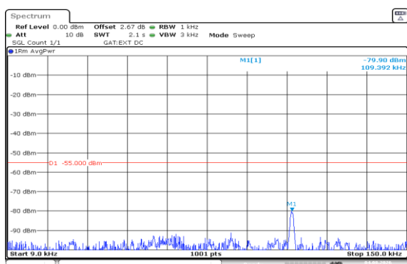
Band41(2535-2655)-20MHz-QPSK-40640-1RB#99-0.009~0.15-PASS
