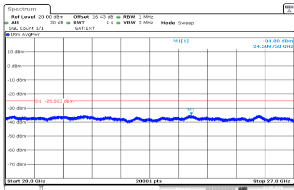
Band41(2535-2655)-20MHz-QPSK-40640-1RB#99-20000~27000-PASS
