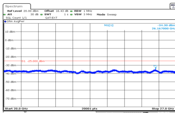
Band41(2535-2655)-20MHz-16QAM-40640-1RB#0-20000~27000-PASS
