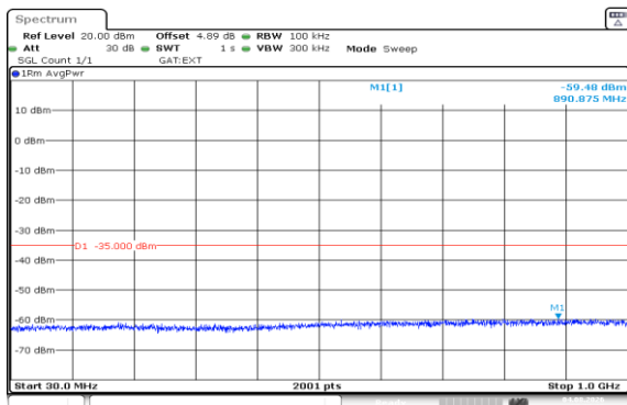
Band41(2535-2655)-20MHz-QPSK-40640-100RB#0-30~1000-PASS
