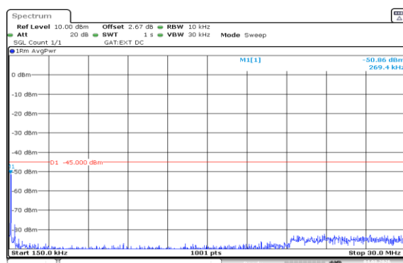
Band41(2535-2655)-20MHz-QPSK-40640-1RB#99-0.15~30-PASS
