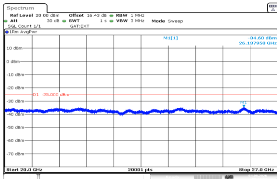
Band41(2535-2655)-20MHz-QPSK-40640-100RB#0-20000~27000-PASS
