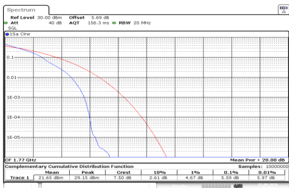
Band66-20MHz-QPSK-132572-1RB#0-PASS
