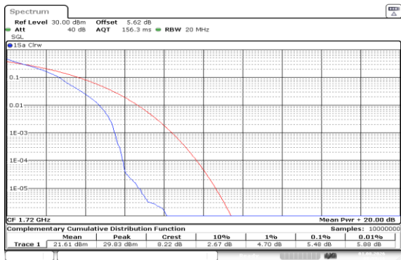
Band66-20MHz-QPSK-132072-1RB#0-PASS
