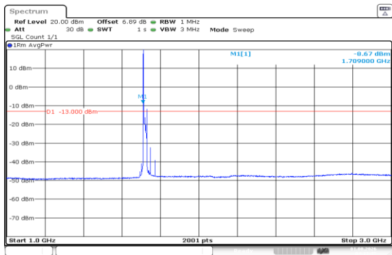
Band66-20MHz-QPSK-132072-1RB#0-1000~3000
