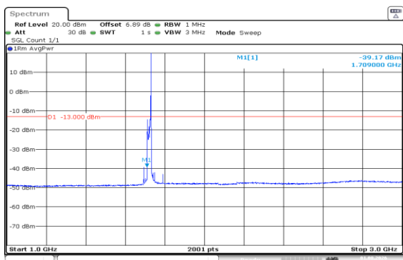
Band66-20MHz-QPSK-132072-1RB#99-1000~3000-PASS
