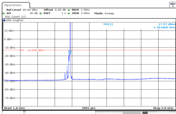
Band66-20MHz-QPSK-132572-1RB#99-1000~3000-PASS
