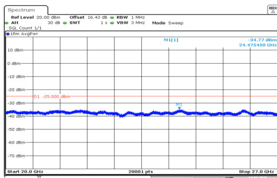
Band7-20MHz-QPSK-20850-100RB#0-20000~27000-PASS
