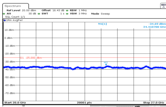
Band7-15MHz-QPSK-20825-1RB#0-20000~27000-PASS
