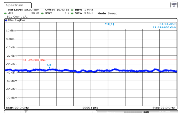
Band7-20MHz-QPSK-21350-100RB#0-20000~27000-PASS
