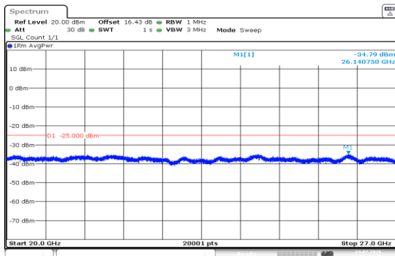
Band7-15MHz-16QAM-20825-1RB#74-20000~27000-PASS
