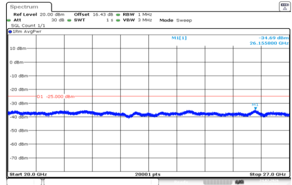
Band7-20MHz-QPSK-20850-1RB#0-20000~27000-PASS
