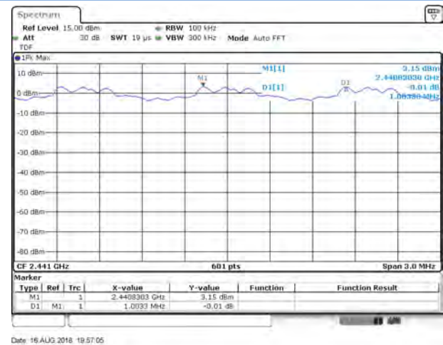
\Pi/4 -DQPSK
