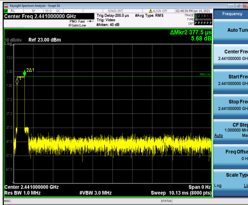
DH1_Ant1_Hop_2441
