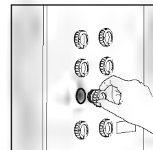
FIG. 3 FUSE BOX
