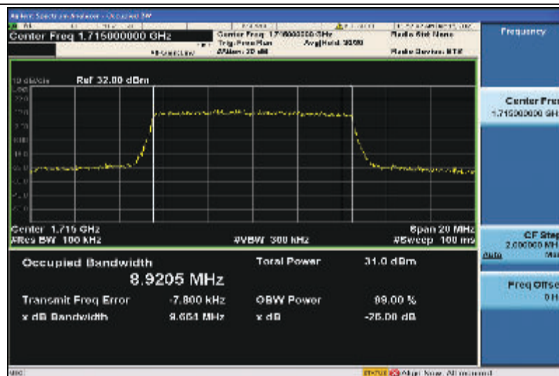
Band4-10MHz-QPSK-20000-50RB#0-8.9205
