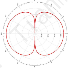
Vertical 3dB beamwidth (°)
