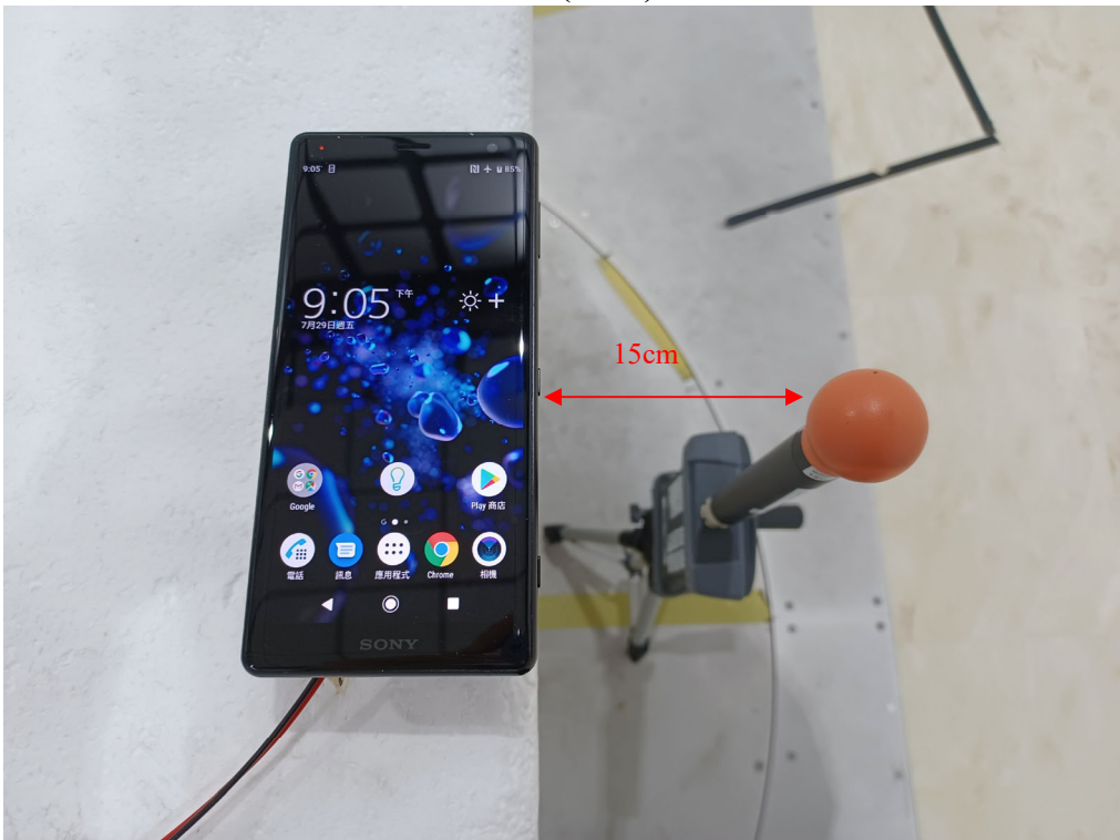
Side 4 (15cm)
