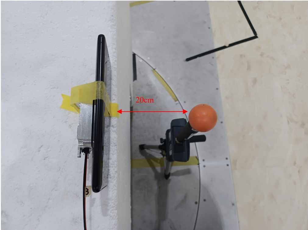
Top (20cm)
