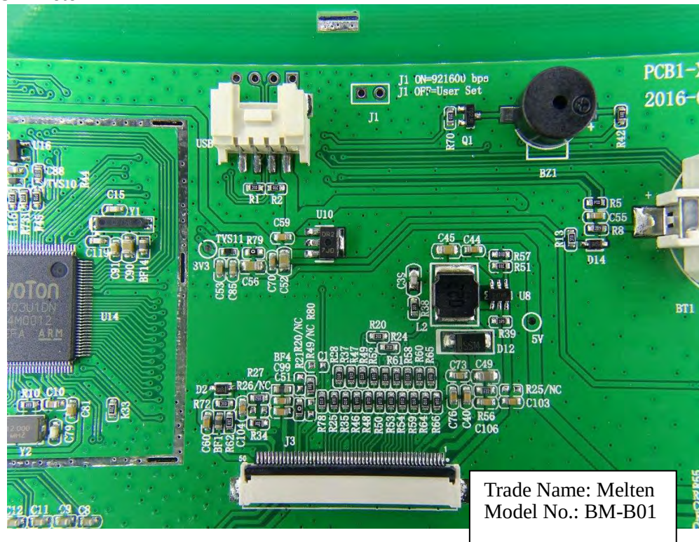
(41) EUT Photo
