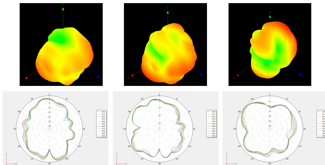
BT 天线增益效率表
