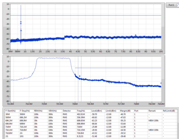
Band 12 LTE 1.4MHz_Nss1,QPSK_1TX 715.3MHz_QPSK_RB 1,#RB H
