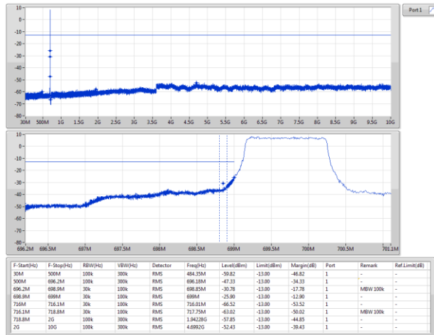
Band 12 LTE 1.4MHz_Nss1,QPSK_1TX 699.7MHz_QPSK_RB 1,#RB 1
