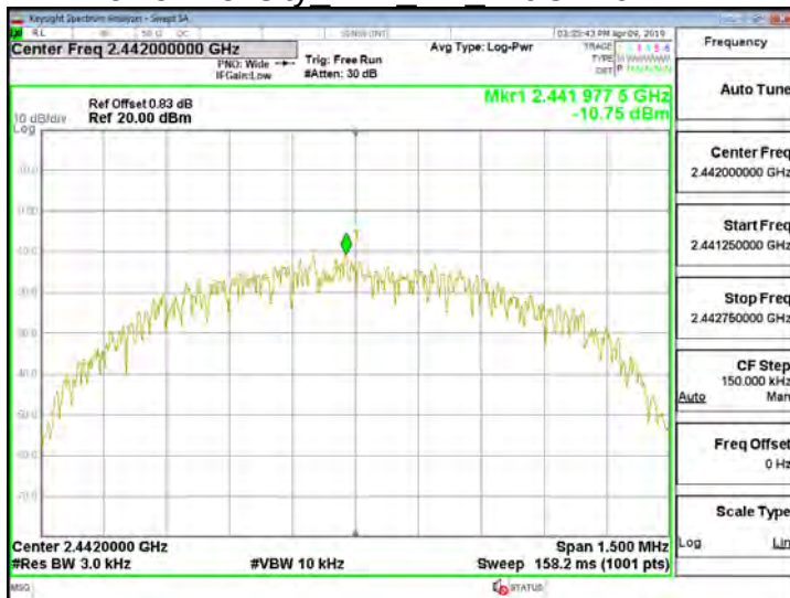
Power Density BLE 1M MidCH19-2442
