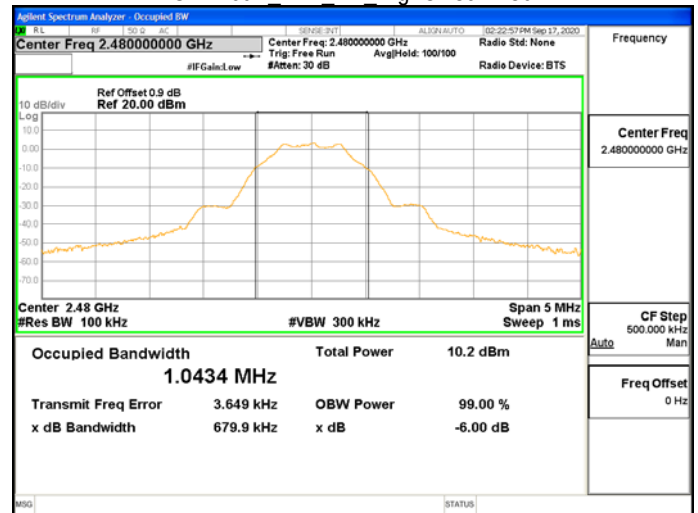
OBW 6dB BLE 1M HighCH39-2480
