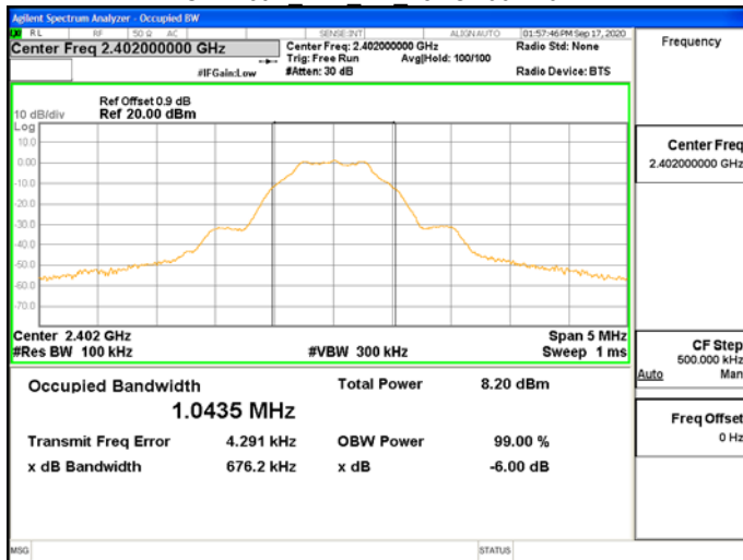
OBW 6dB BLE 1M LowCH00-2402
