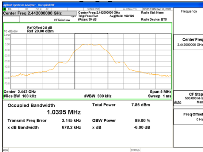
OBW 6dB BLE 1M MidCH20-2442
