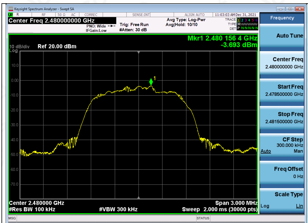
Test_Graph_EDR_ANT1_2480_3Mbps_Reference Level
