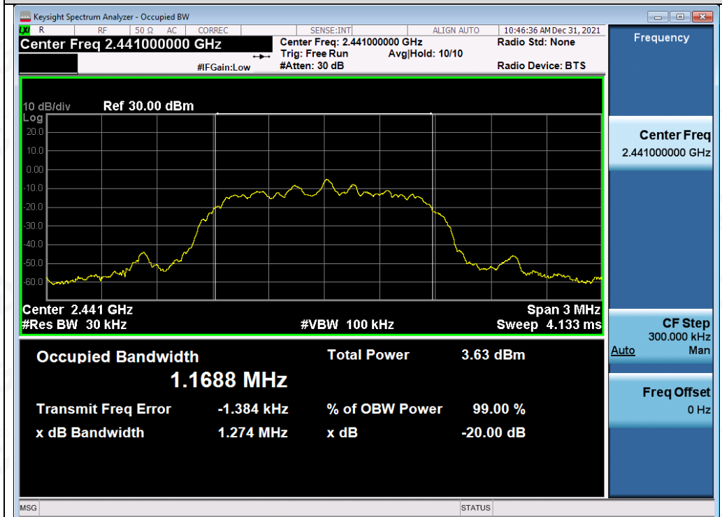
Test_Graph_EDR_ANT1_2441_2Mbps_OBW
