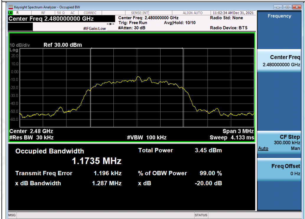
Test_Graph_EDR_ANT1_2480_3Mbps_OBW
