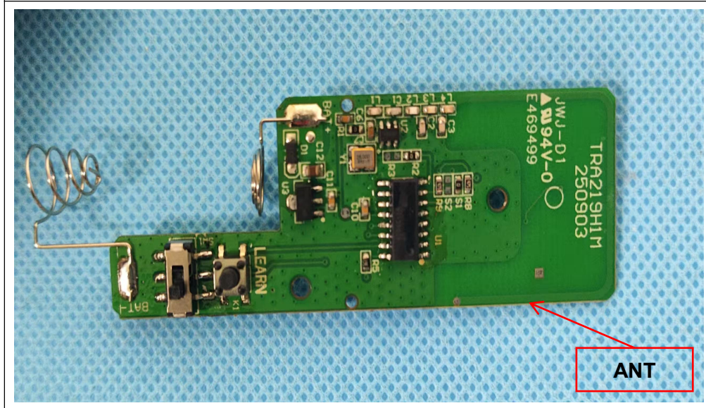
ANT
