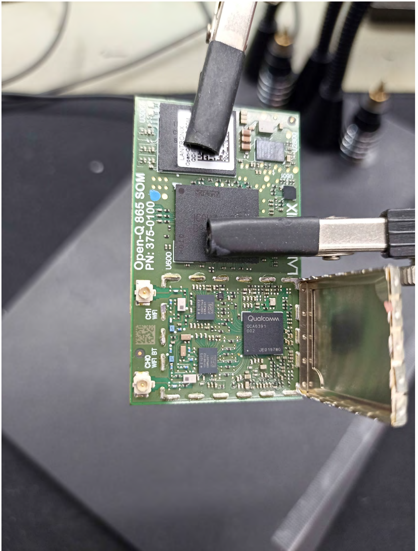
RF Module Top Side The SoM with the shield removed
