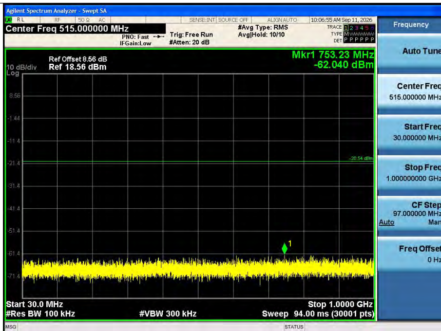
BLE 2M Ant1 2478 30~1000
