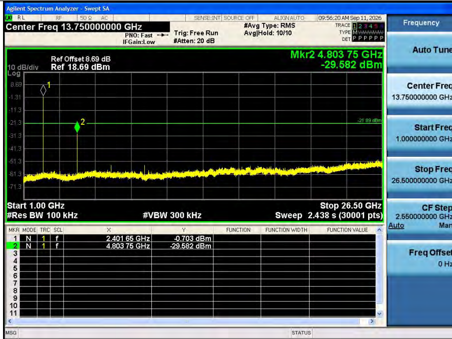
BLE 1M Ant1 2402 1000~26500
