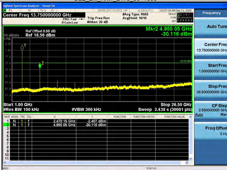
BLE 2M Ant1 2478 1000~26500
