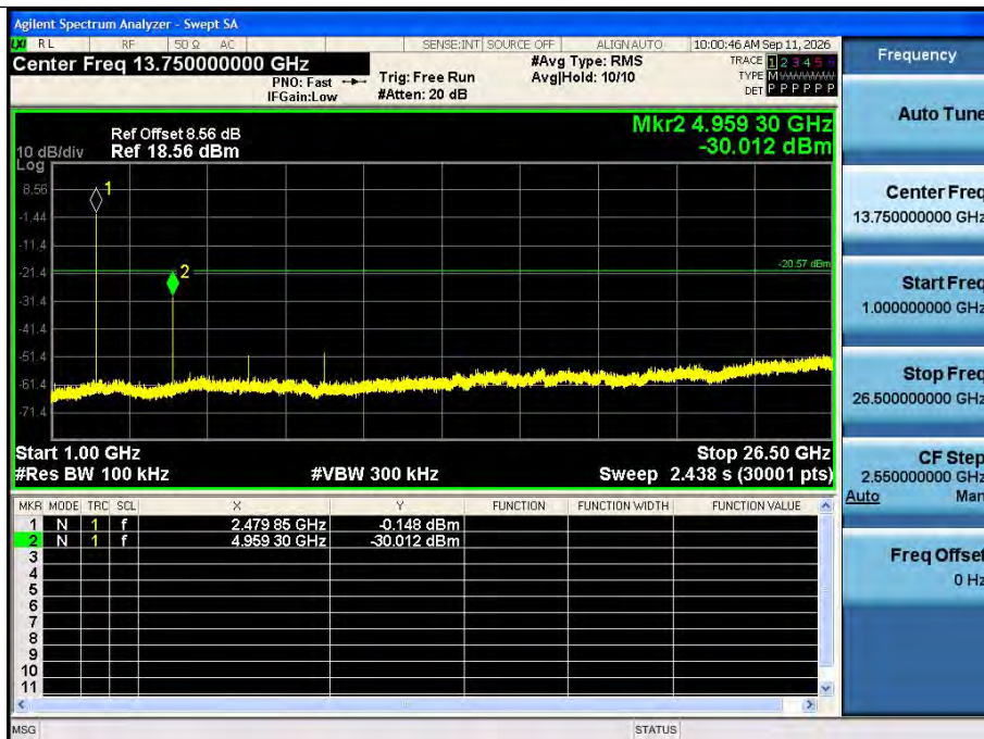
BLE 1M Ant1 2480 1000~26500
