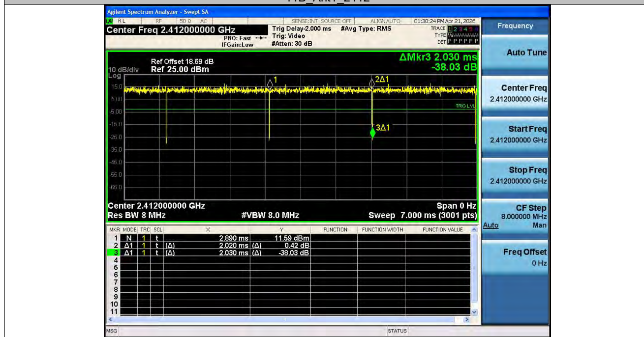
11G Ant1 2412
