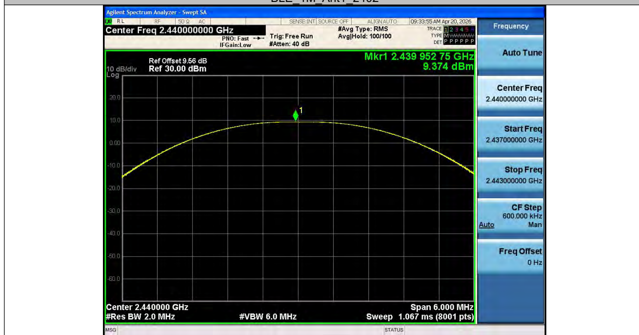
BLE_1M Ant1 2440
