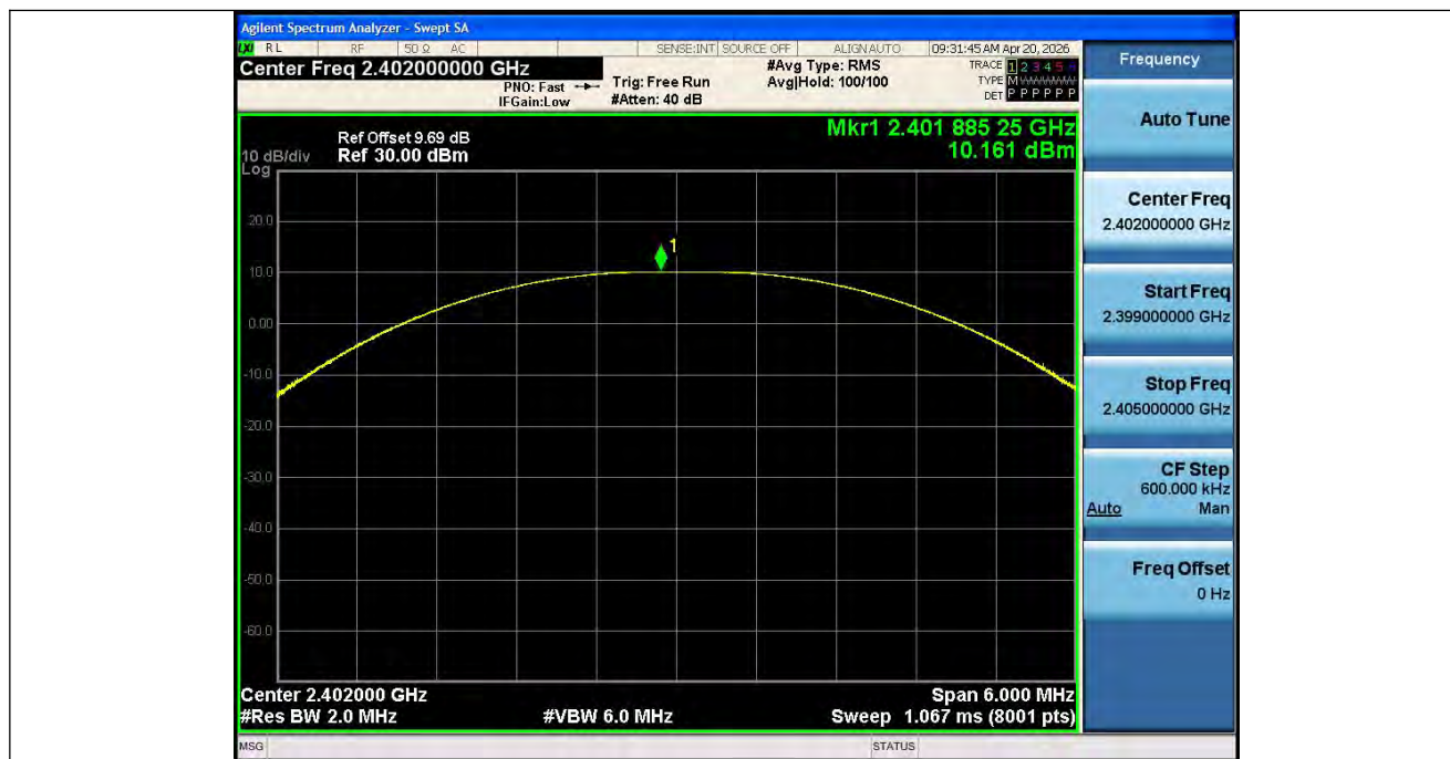
BLE_1M Ant1 2402
