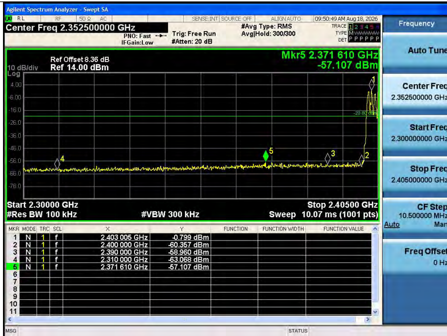
DH5 Ant1 Low Hop 2402
