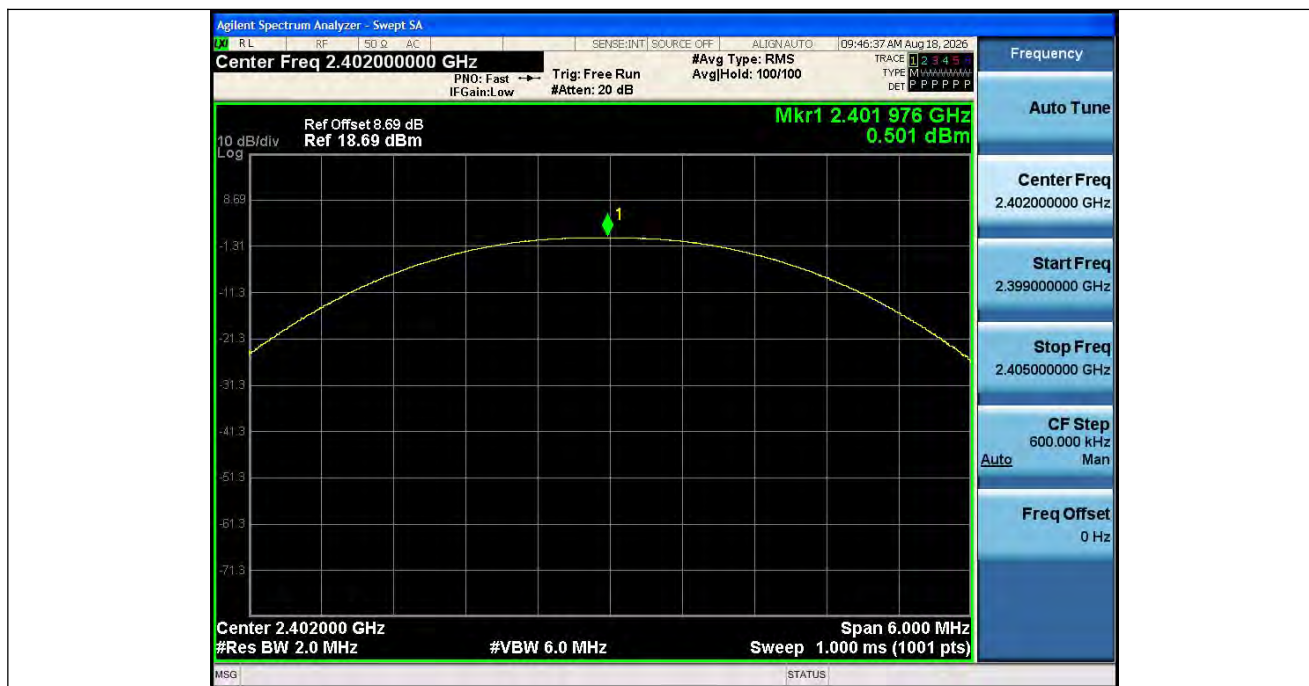
DH5_Ant1_2402
