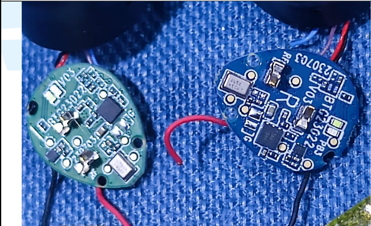
EUT Photo
