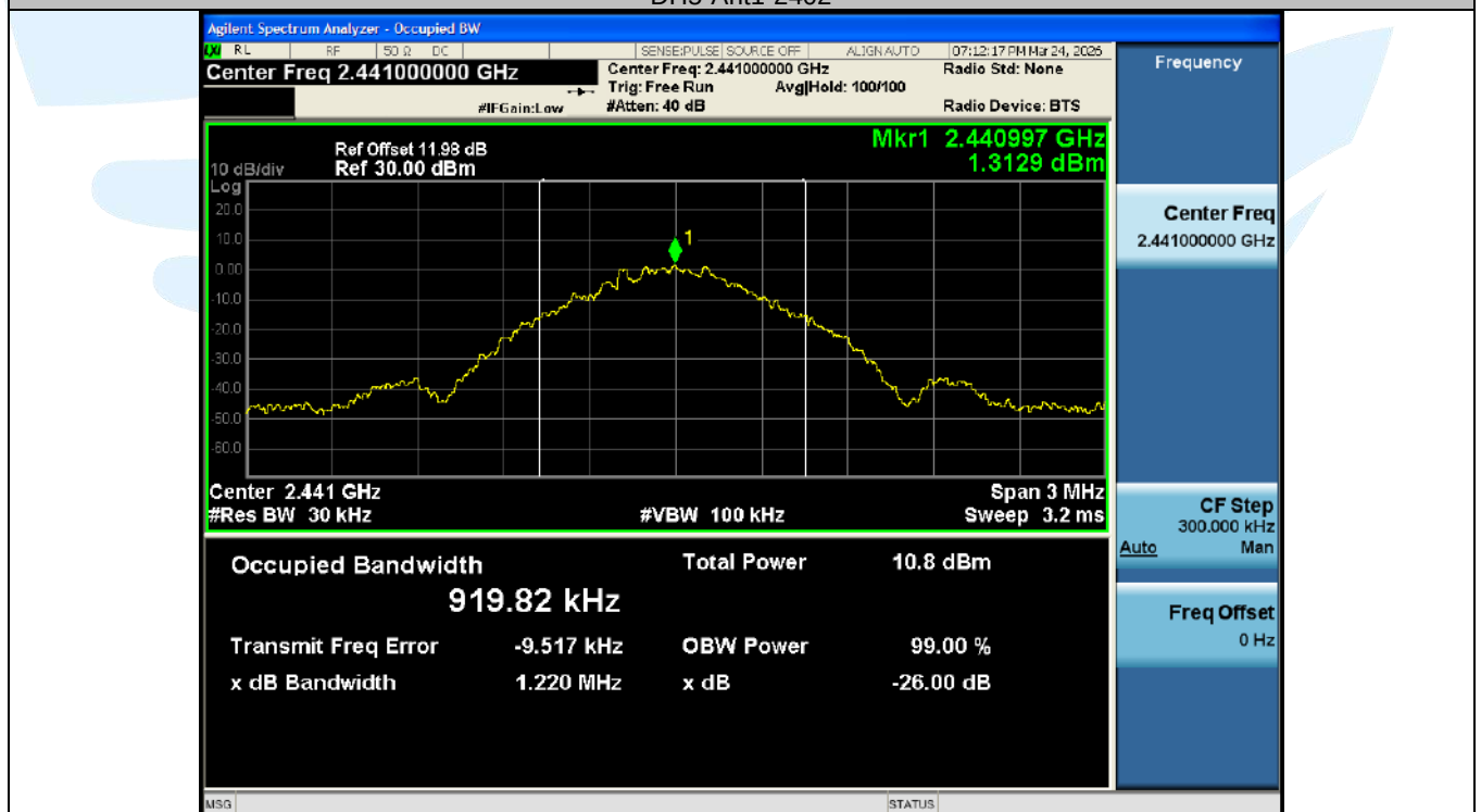
DH5-Ant1-2441
