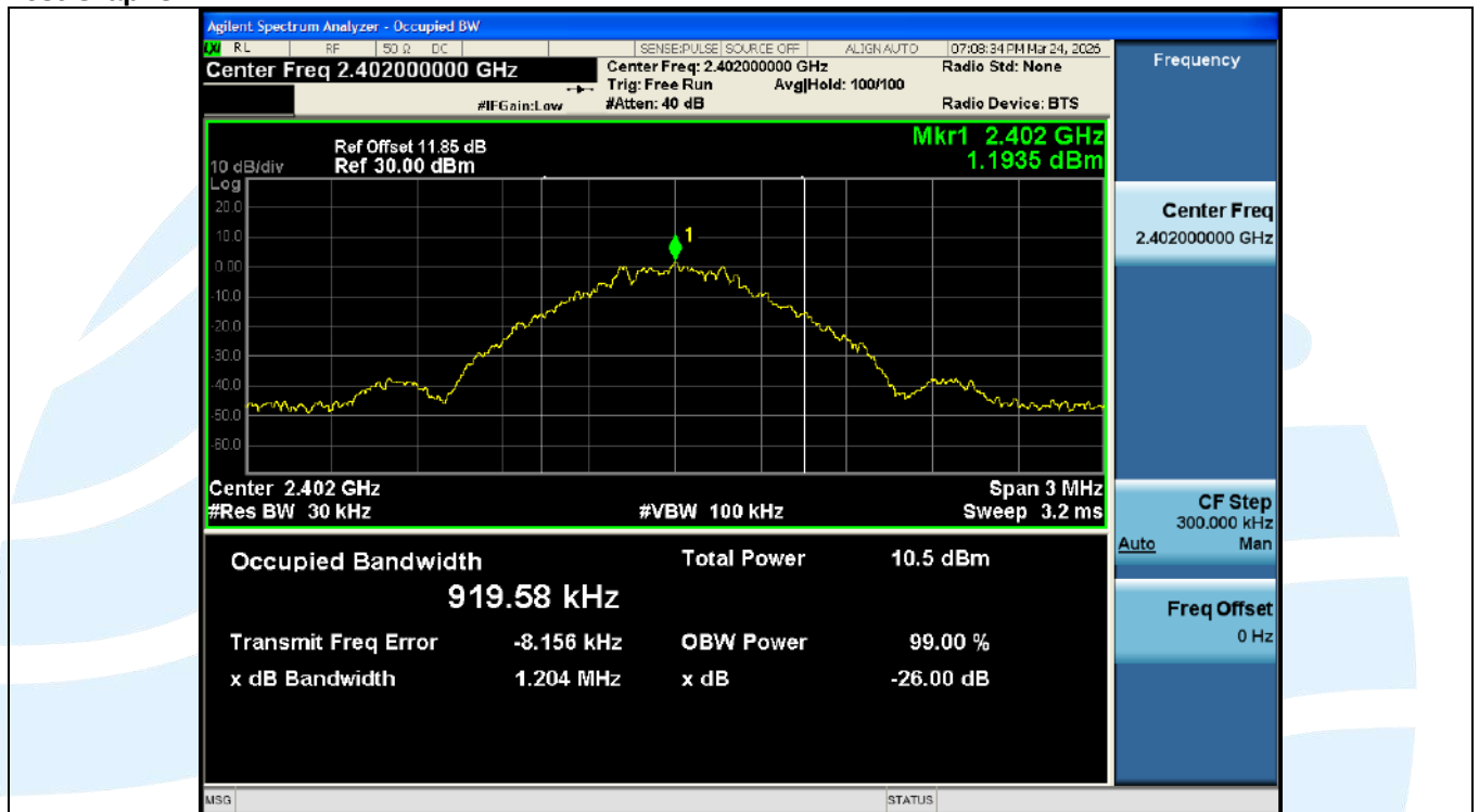
DH5-Ant1-2402
