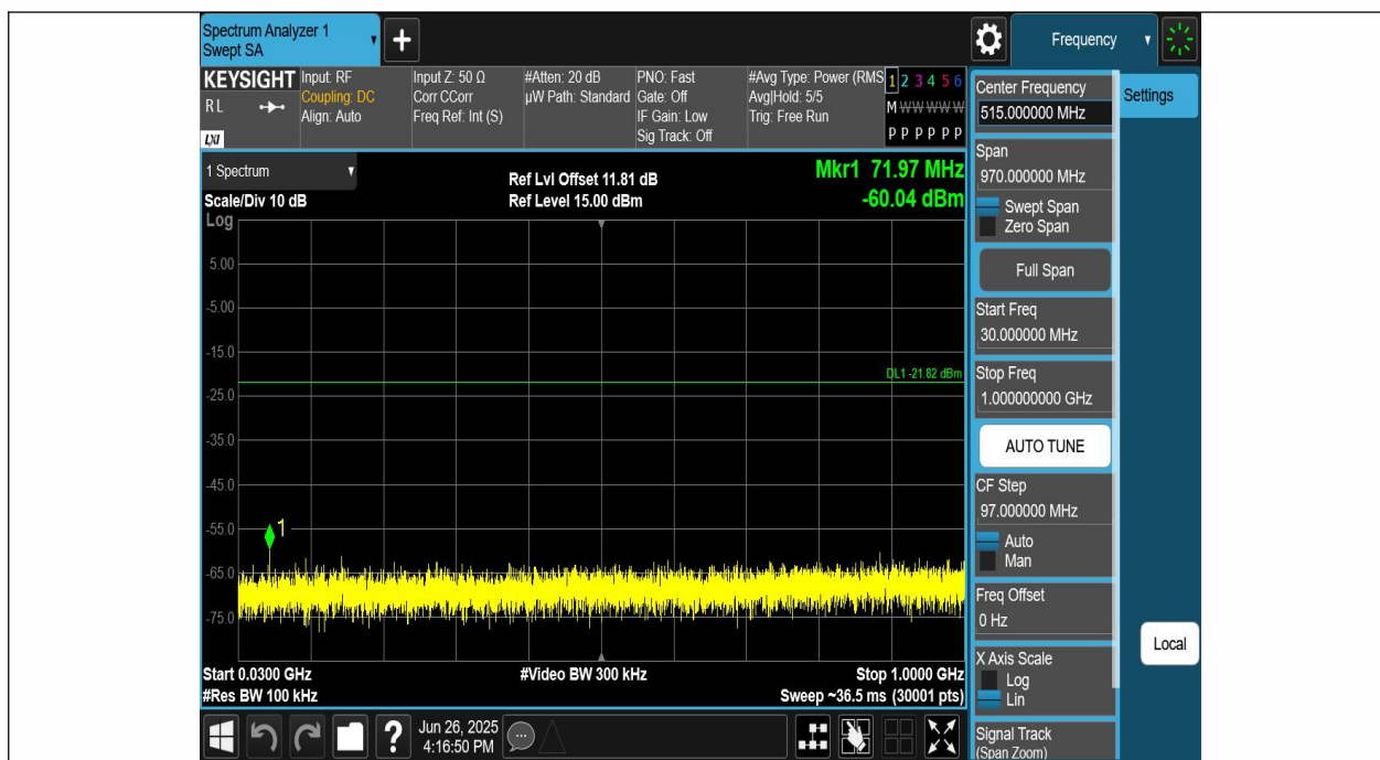
BLE_2M-Ant1-2402-30~1000-PASS
