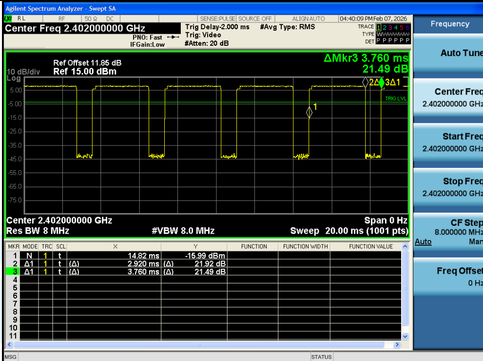
NTNV-2DH5-Ant1-2402
