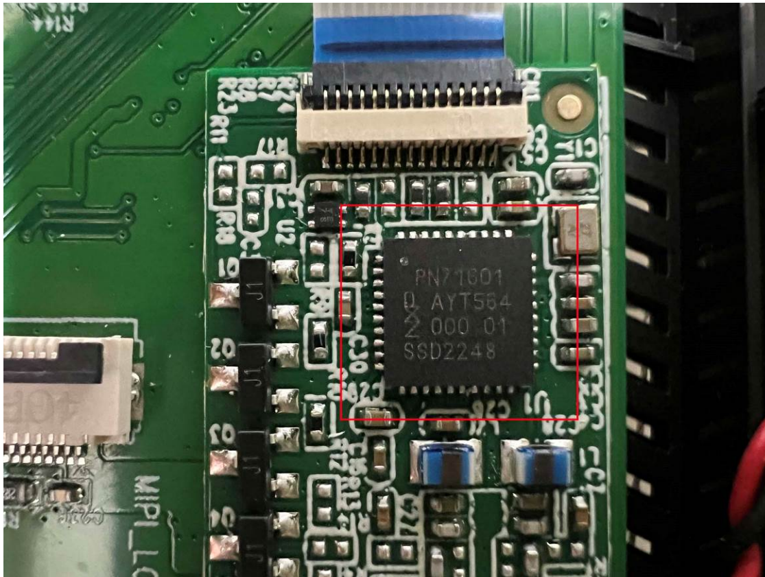
EUT-5. Module PN7160
