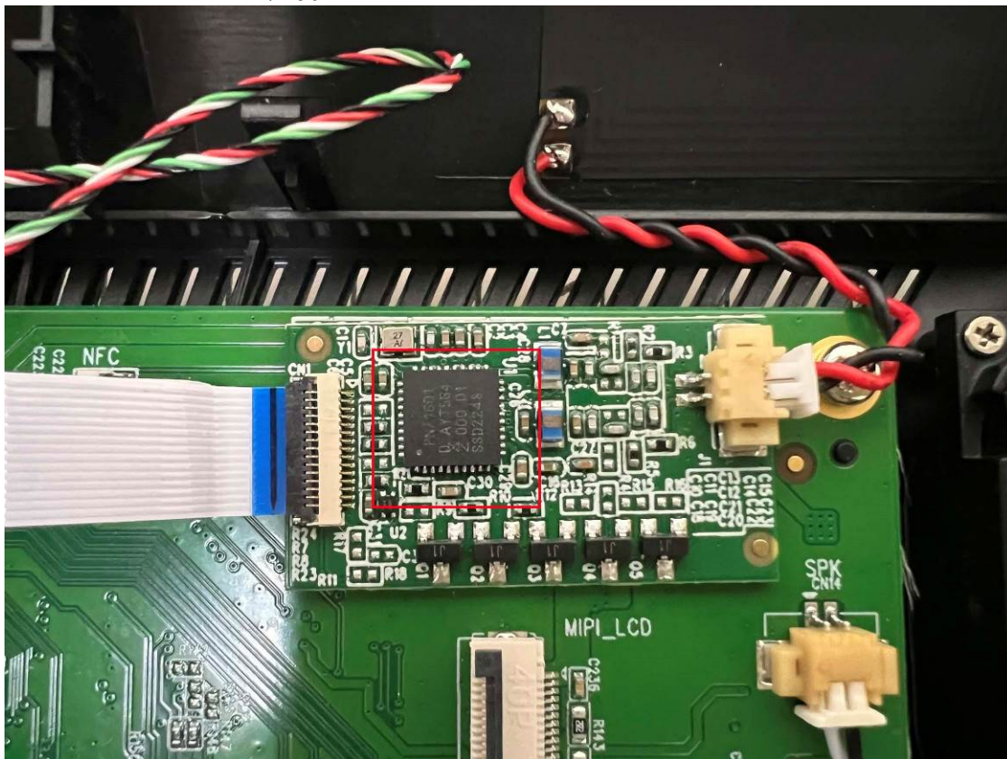
EUT-4. Module PN7160
