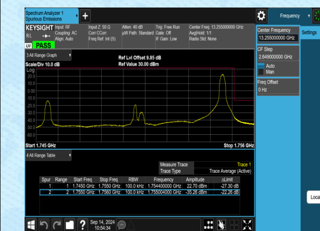
Band4-10MHz-QPSK-20350-1RB#49-PASS
