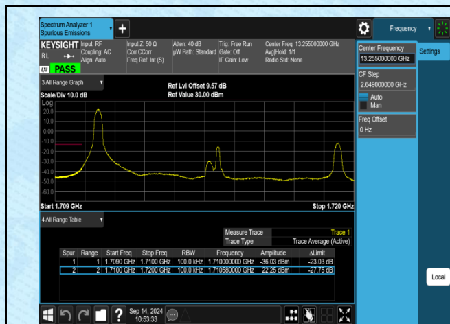
Band4-10MHz-QPSK-20000-1RB#0-PASS
