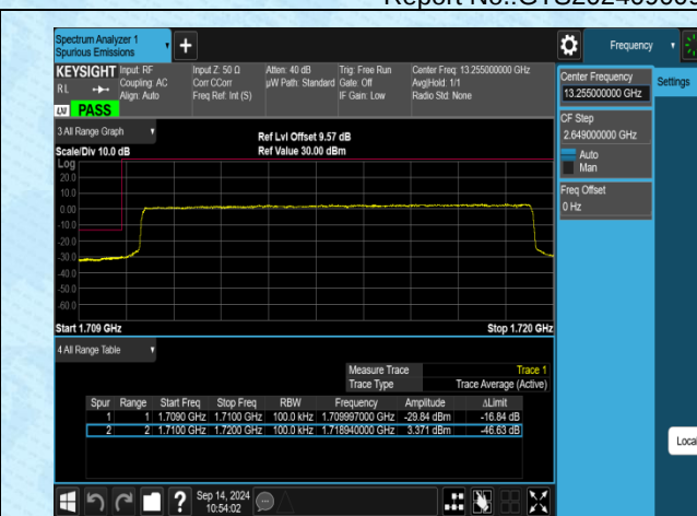
Band4-10MHz-QPSK-20000-50RB#0-PASS
