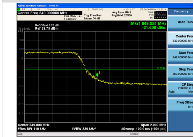
HCH_QPSK_25RB#0
