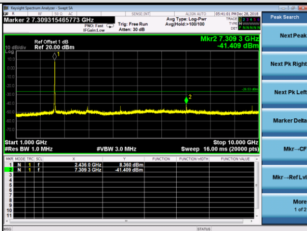
11B-MCH
