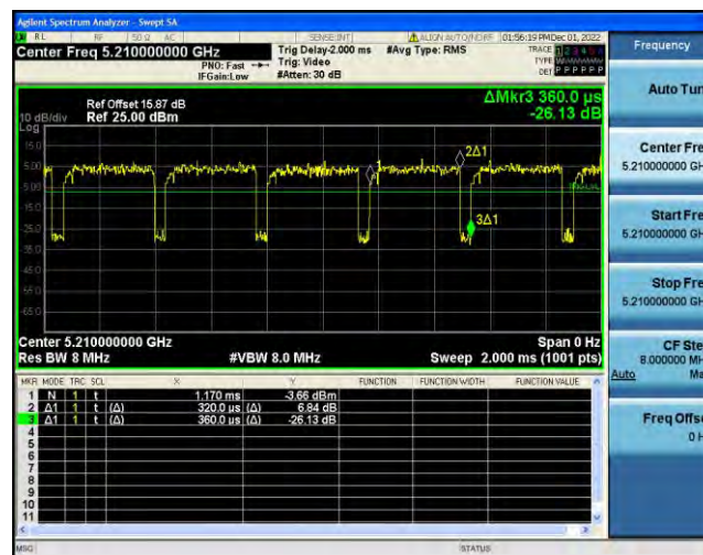
NTN-11AC80SISO-Ant2-5210-0.33-0.37
