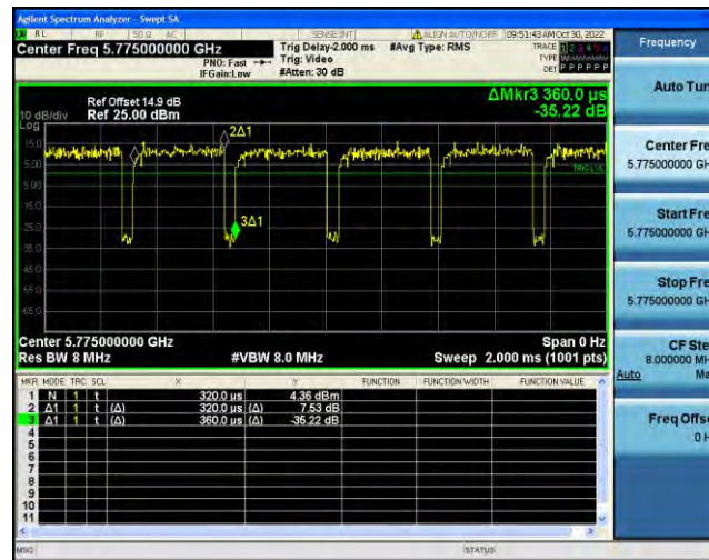
NTNV-11AC80SISO-Ant2-5775-0.32-0.36
