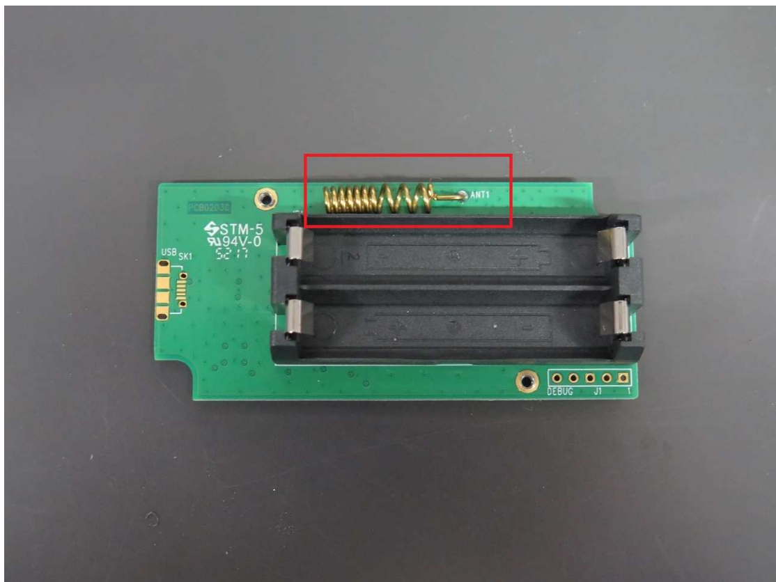
Door Sensor (EUT antenna)
