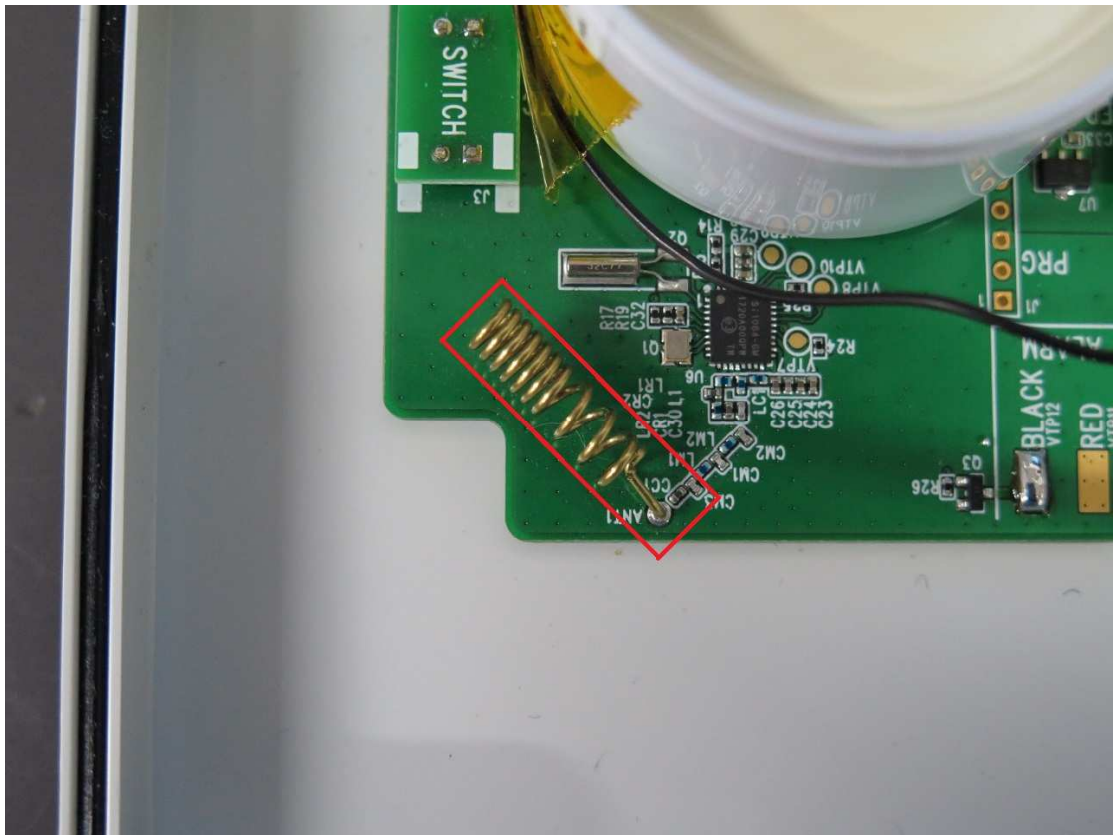
(EUT antenna)
