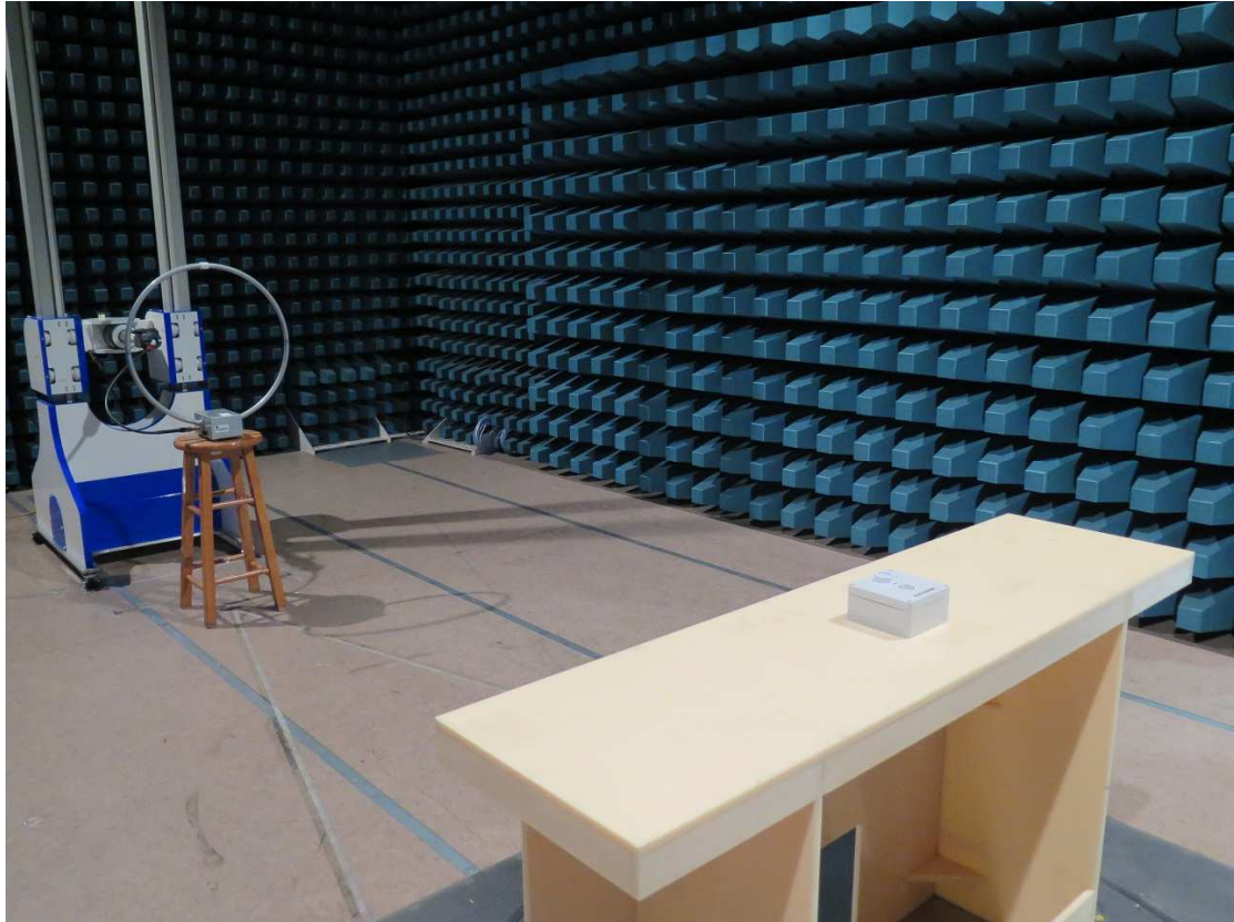
9kHz – 30MHz
