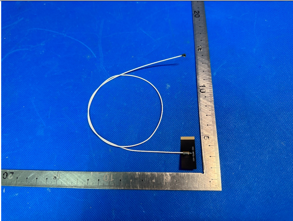
EUT Photo(10) LG-NA-65:N12-8965-R0A
