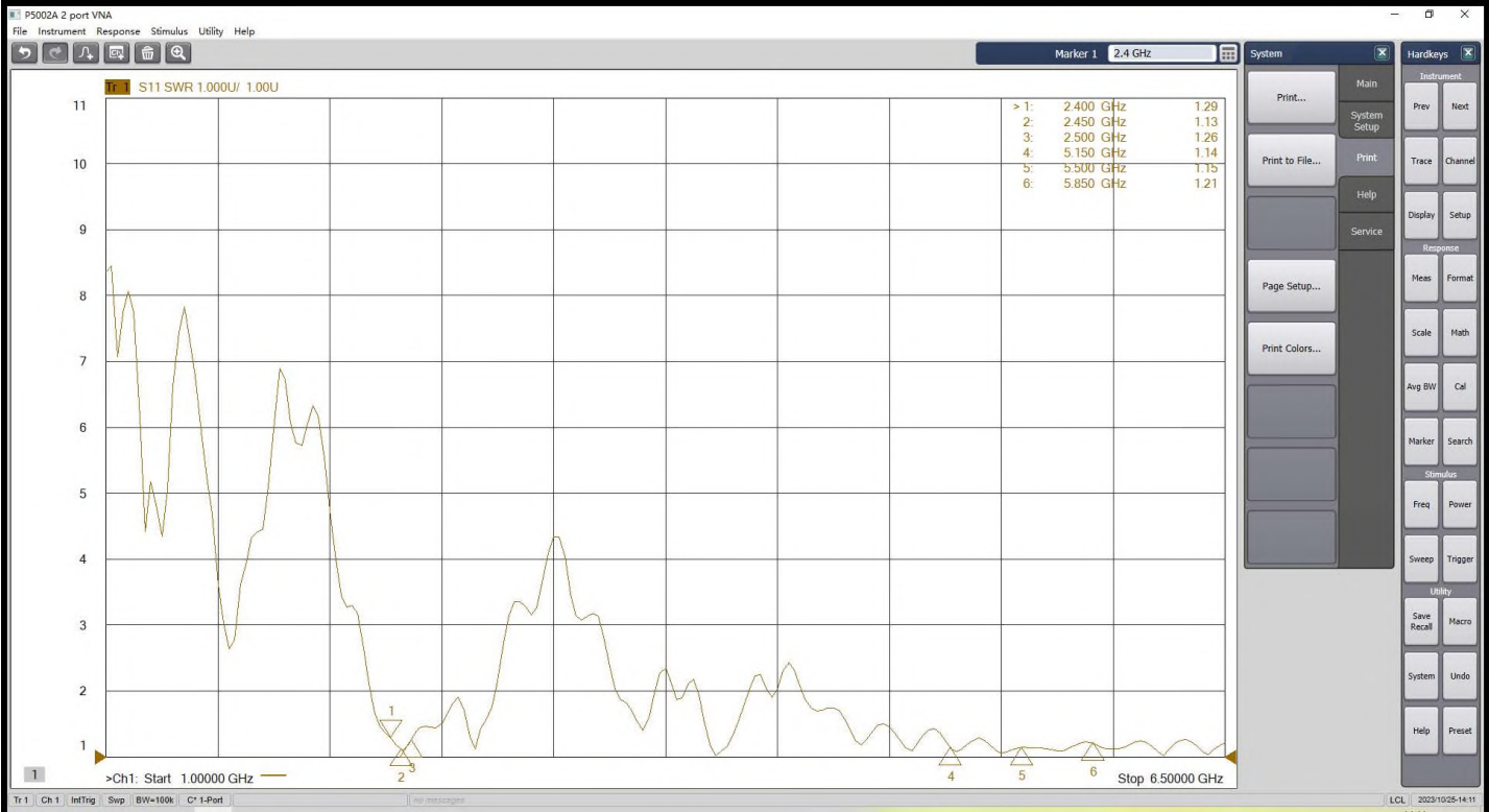
VSWR图
